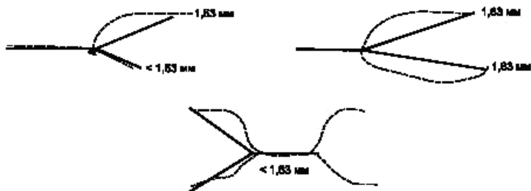
Рисунок F.17 — Методы определения окончания ветвей
