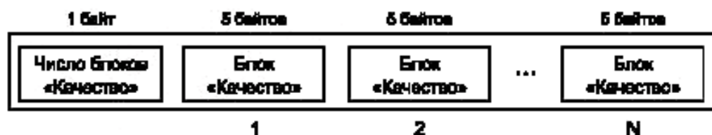
Рисунок 6 — Диаграмма блоков «Качество» изображения отпечатка пальца
