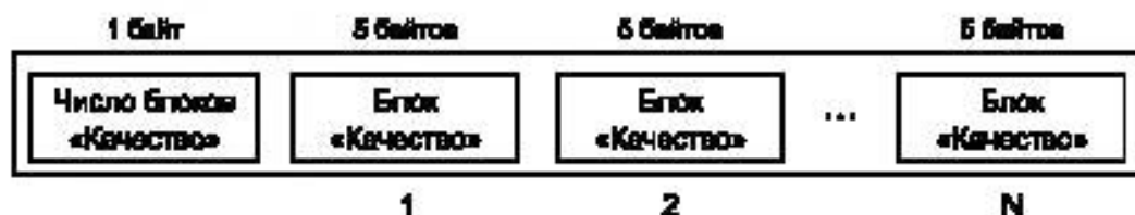
Рисунок 6 — Диаграмма блоков «Качество» изображения отпечатка пальца
