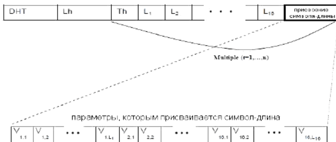
Рисунок E.14 – Синтаксическая структура спецификации таблицы Хаффмана
