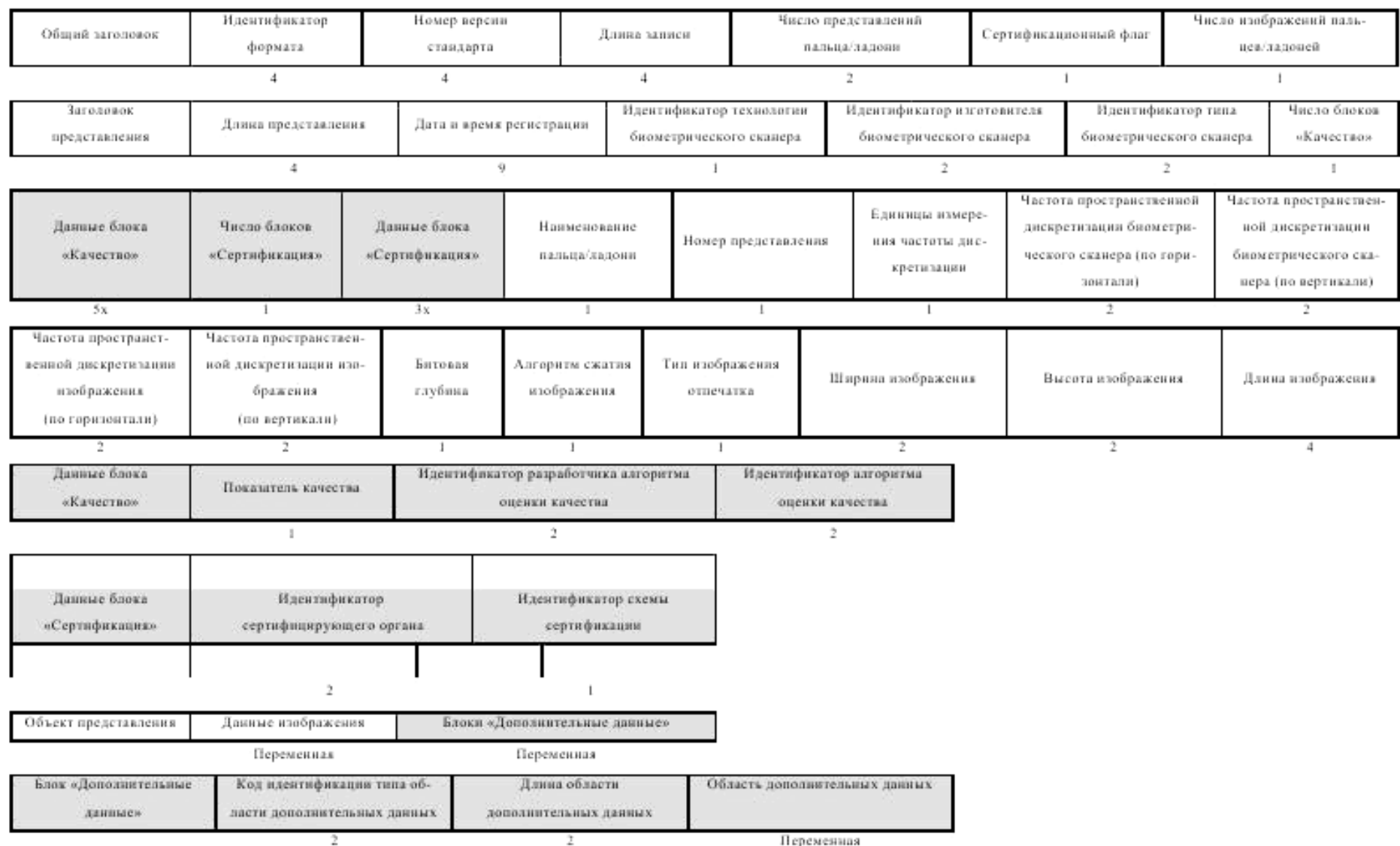
Рисунок 3 – Порядок расположения и размер полей записи изображения отпечатка пальца
