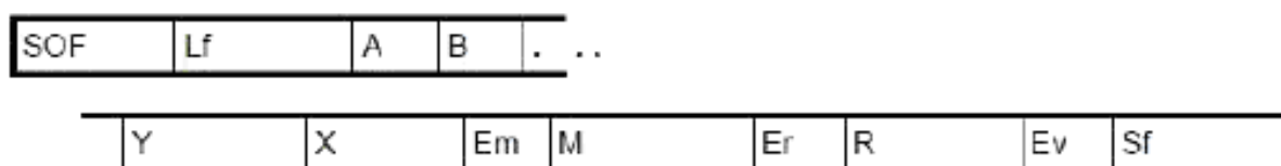
Рисунок E.9 – Синтаксическая структура заголовка кадра
