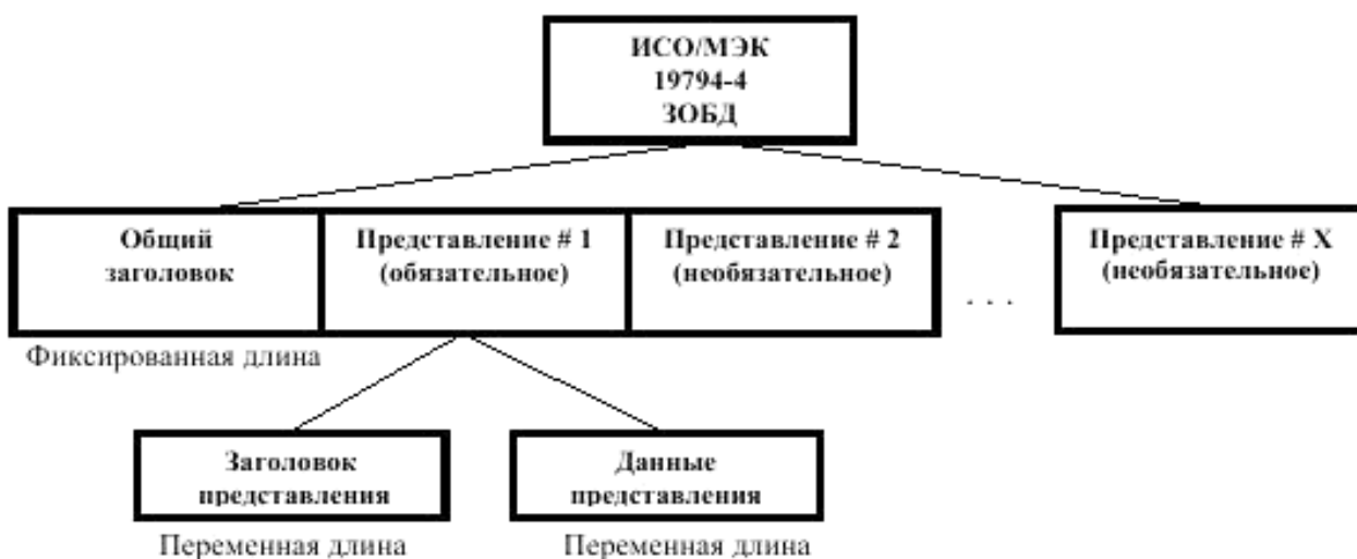
Рисунок 2 – Структура формата записи изображения отпечатка пальца
