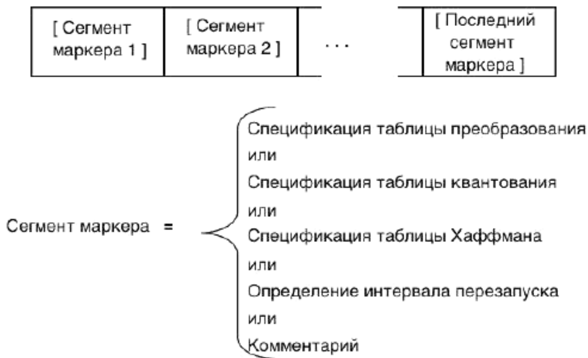
Рисунок Е.11 – Синтаксическая структура табличных/разных сегментов с маркерами
