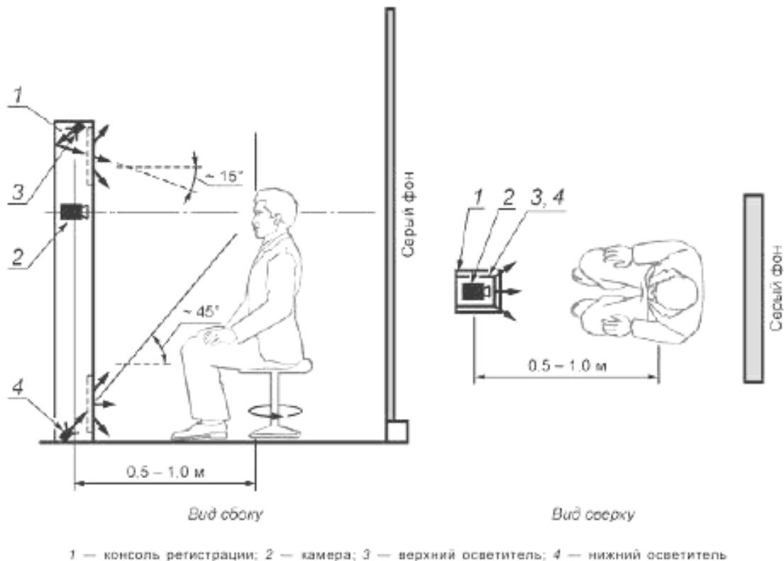
Рисунок С.10 — Рекомендации для взаиморасположения субъекта, камеры и источников освещения в пункте регистрации
