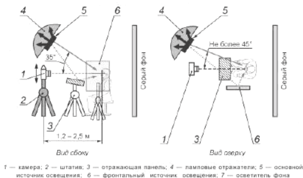
Рисунок С.6 — Организация освещения в фотолаборатории с использованием двух источников освещения и осветителя фона
