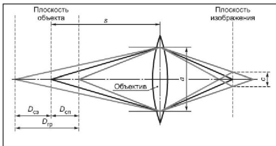
Рисунок С.1 — Параметры для вычисления глубины поля
