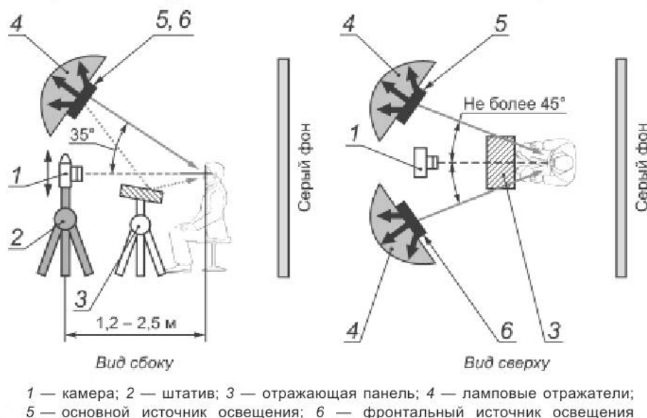
Рисунок С.5 — Организация освещения в фотолаборатории с использованием двух источников освещения
