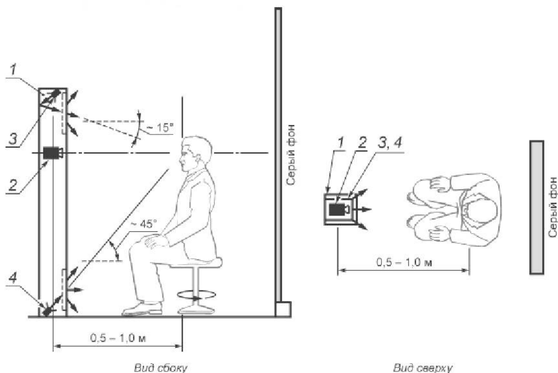
1 — консоль регистрации; 2 — камера; 3 — верхний осветитель; 4 — нижний осветитель
