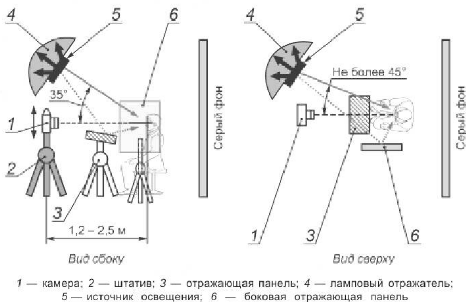
Рисунок С.4 — Организация освещения в фотолаборатории с использованием одного источника освещения
