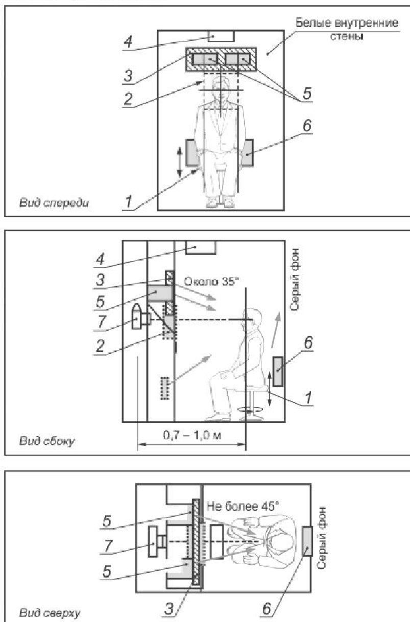
Рисунок С.7 — Рекомендации для взаиморасположения субъекта, камеры и источников освещения в фотокабине
