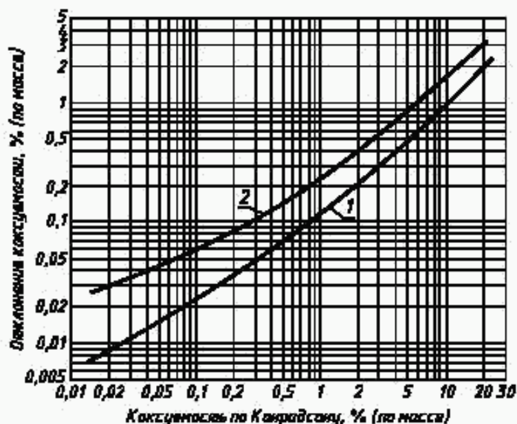
Рисунок 2 — Точностные характеристики
