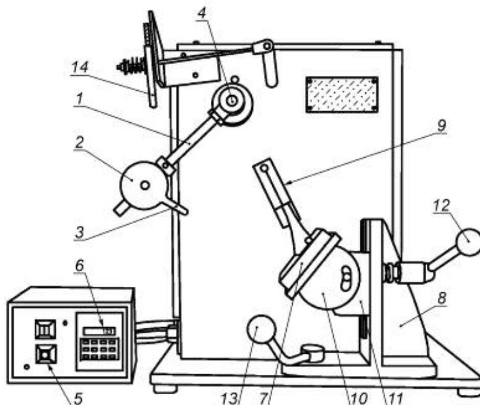
1 — маятник; 2 — груз маятника; 3 — головка бойка; 4 — стул; 5 — выключатель электрического питания; 6 — счетчик; 7 — держатель образца для испытаний; 8 — вертикальная установочная плита; 9 — направляющая пластина, используемая при установке каблук; 10 — основной зажим для ориентации вращения; 11 — зажим для вертикальной ориентации; 12 — устройство для регулировки расположения зажимов 10 и 11 относительно вертикальной установочной плиты 8; 13 — устройство для регулировки в горизонтальной плоскости; 14 — амортизатор обратного хода
