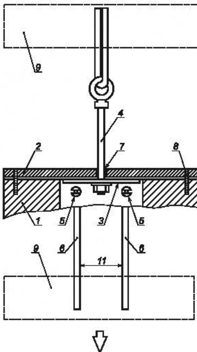
Рисунок 2а — Вид сбоку на испытываемый узел и вертикальный разрез каблука с набойкой
