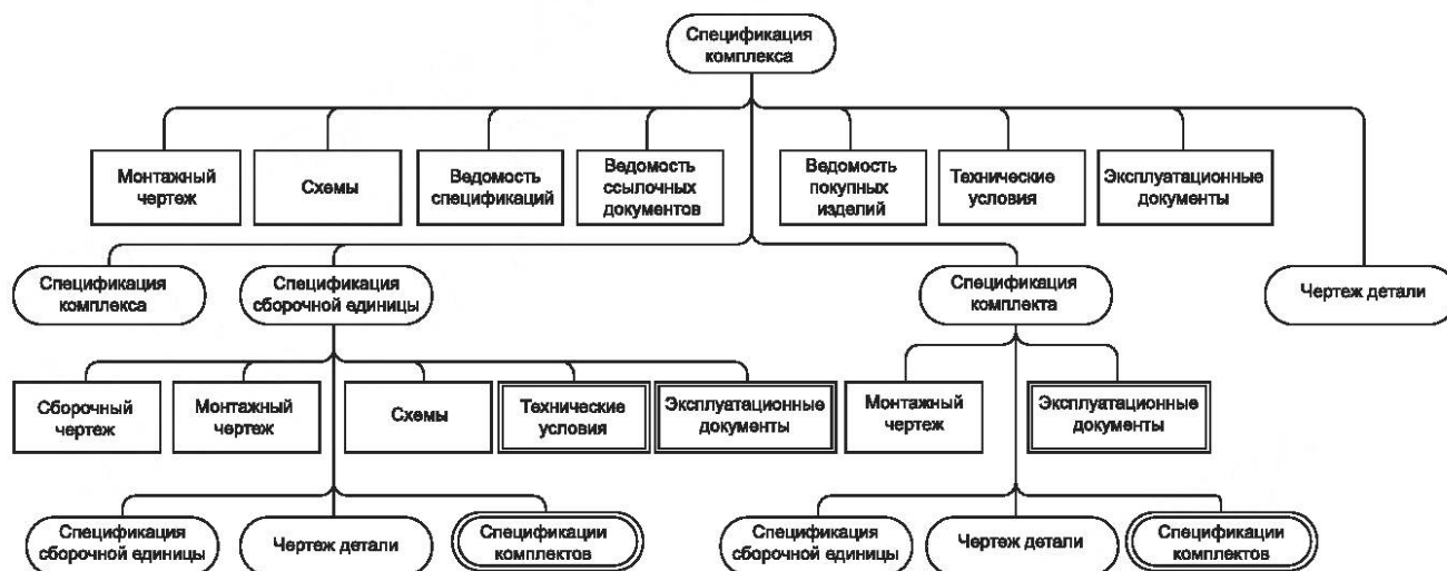
Схема построения полного комплекта конструкторских документов с использованием спецификации
