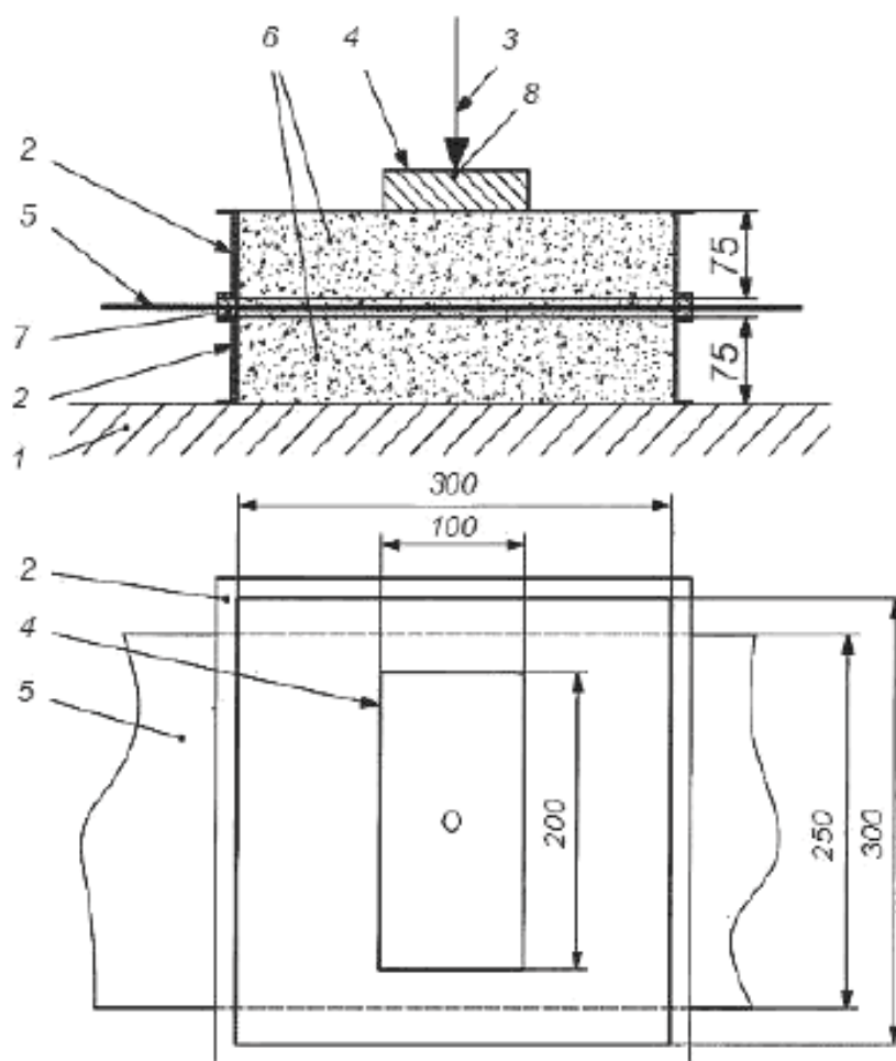
1 — массивное основание; 2 — испытательная форма; 3 — прикладываемая нагрузка; 4 — нагрузочная плита; 5 — испытуемый образец; 6 — дискретный заполнитель; 7 — прокладки; 8 — сферическое гнездо
