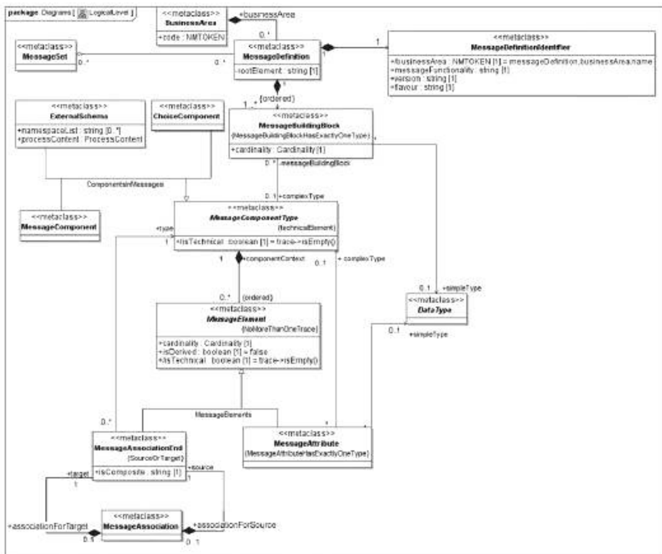
Рисунок 7 — Логический уровень
