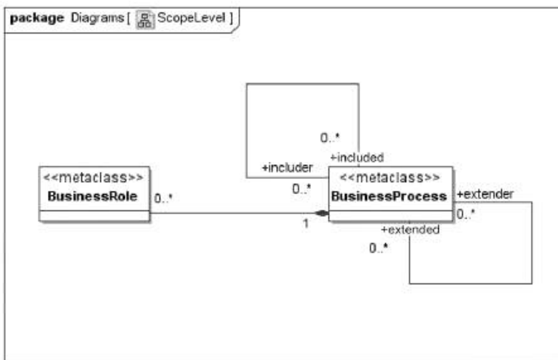
Рисунок 4 — Обзорный уровень
