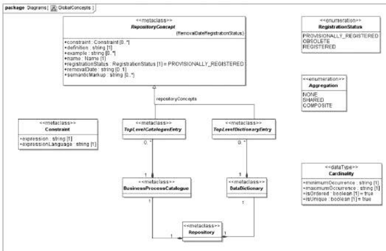
Рисунок 13 — Глобальные концепты
