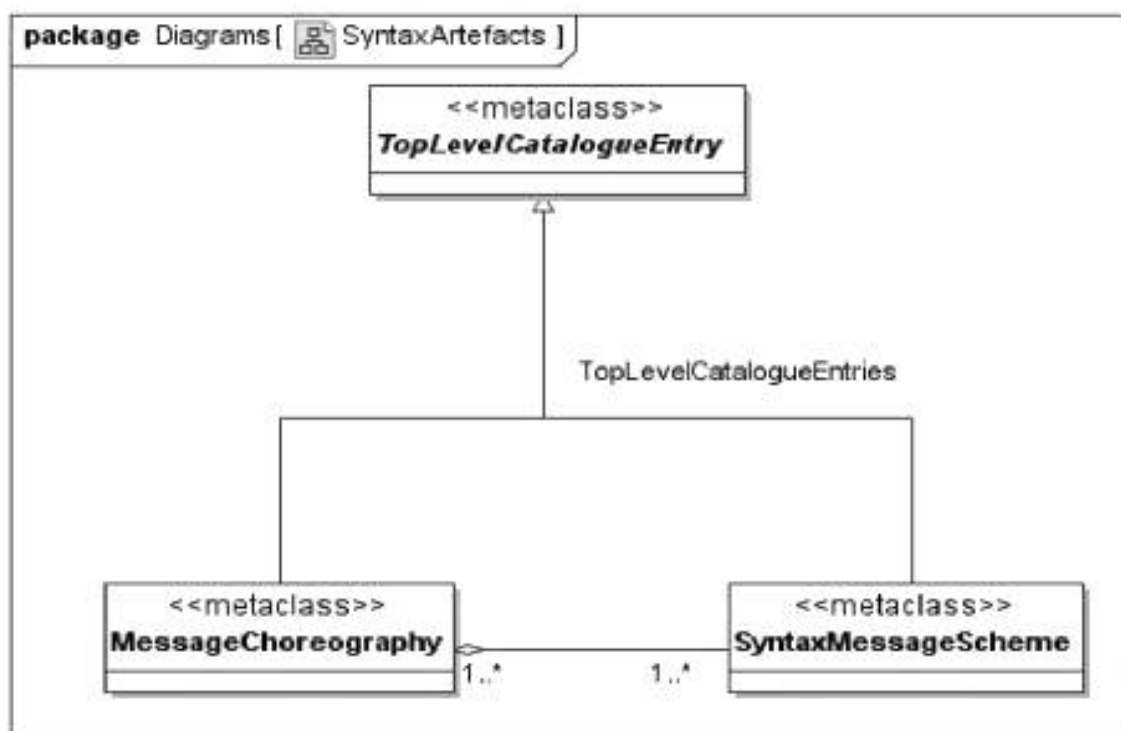
Рисунок 8 — Синтаксис артефактов
