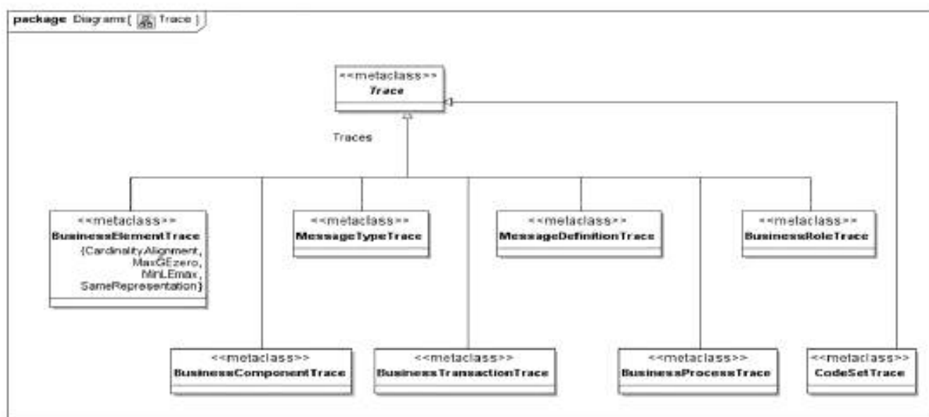
Рисунок 9 — Следы
