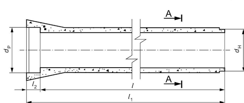
Рисунок А.3 — Общий вид труб типа БТС
