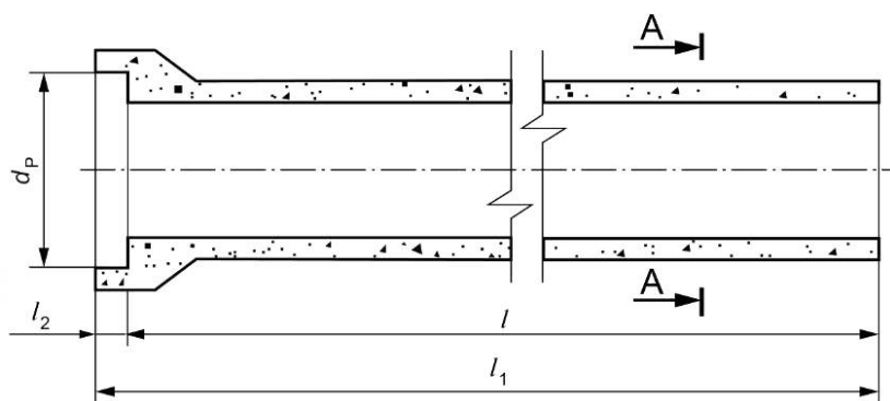
Рисунок А.1 — Общий вид труб типа БТ
