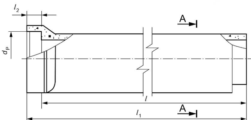
Рисунок А.2 — Общий вид труб типа БТП
