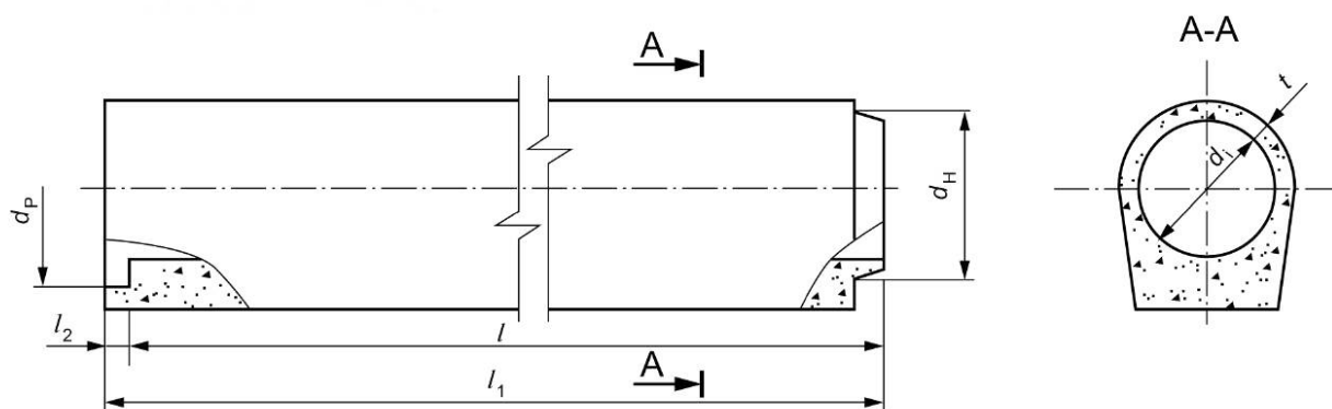
Рисунок А.6 — Общий вид труб типа БТП
