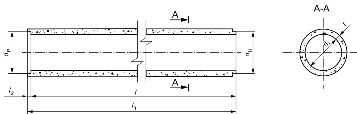
Рисунок А.5 — Общий вид труб типа БТФ
