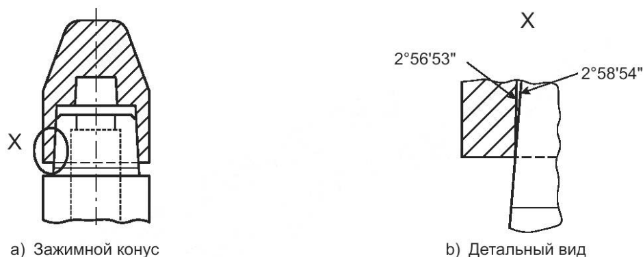
Рисунок 1 — Принцип работы зажимного конуса
