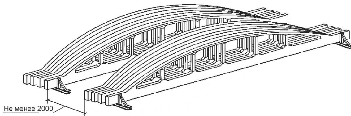
Рисунок 1 — Складирование ферм
