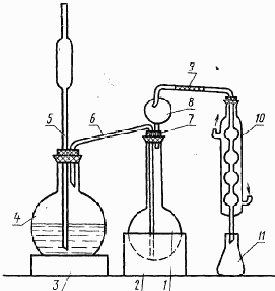
Прибор для перегонки водяным паром
