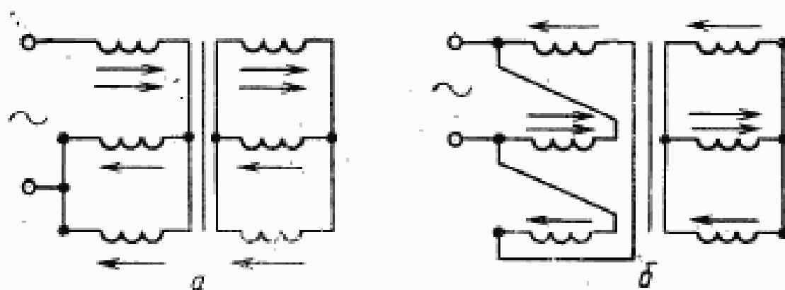
Двумя стрелками обозначена испытываемая фаза, по которой протекает ток КЗ вдвое больший, чем в двух других фазах.
