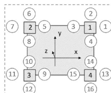
Рисунок С.4 — Иллюстративный материал к примеру 3 (квадратами с цифрами изображены упругие опоры, кружочками с цифрами — акселерометры в точках контроля)
