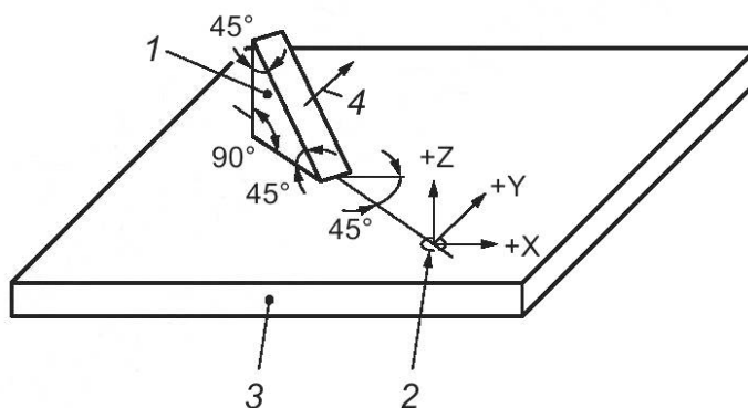
Рисунок D.1 — Схематическое изображение испытательной установки для измерений затормаживающих сил в области контакта между источником вибрации и приемной конструкцией
