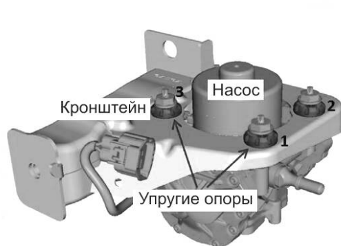
а) Насос/источник, соединенный с кронштейном/приемником через три упругие опоры/точки контакта
