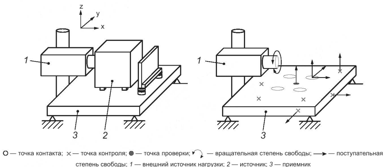
Рисунок С.1 — Графическое изображение сборки, нагрузки и направлений движения
