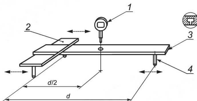
Рисунок А.1 — Пример устройства для измерения плоскостности по ширине
