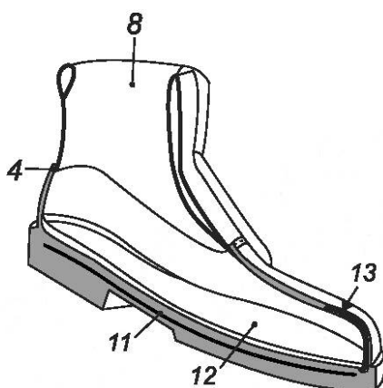
а) Пример комбинированной защитной обуви в общем случае
