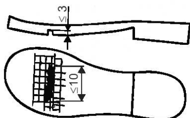
д) Трещины в подошве
