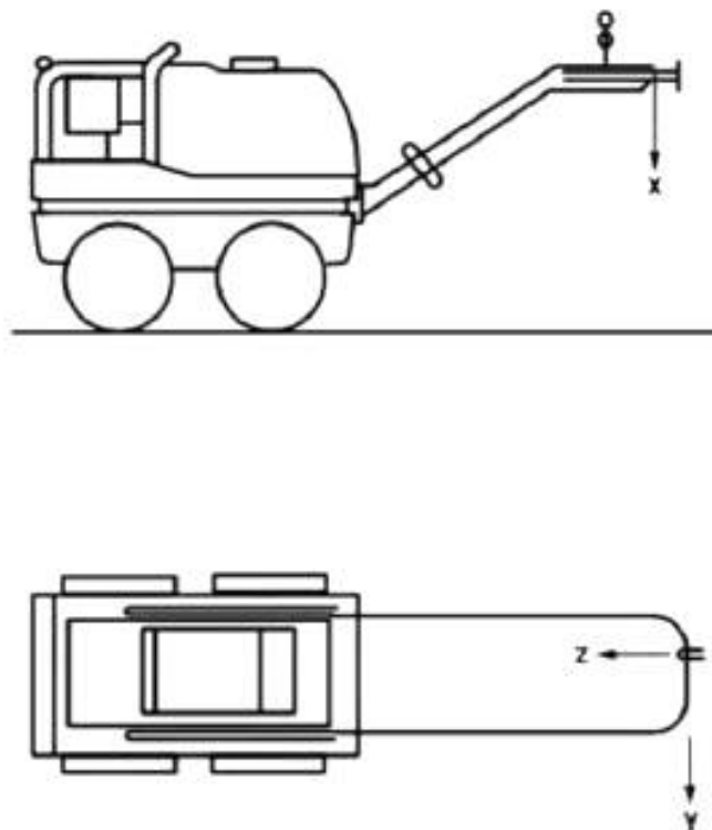
Рисунок В.1 – Направления измерений
