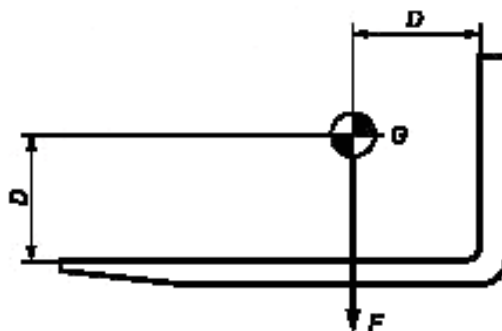
Рисунок 1 — Расстояние центра тяжести нагрузки
