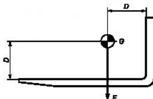
Рисунок 1 — Расстояние центра тяжести нагрузки
