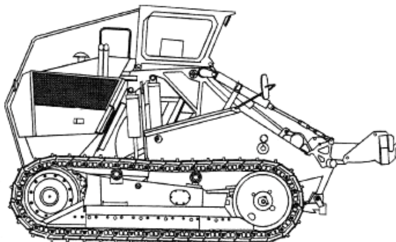
Рисунок А.4 — Гусеничный скрепер
