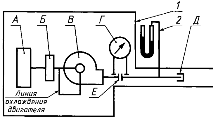
СХЕМА ИСПЫТАНИЯ УСТАНОВОК ФВУ А (внутреннее размещение)
