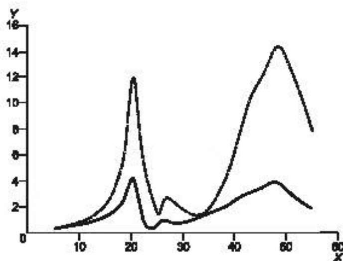
X — частота, Гц; Y — среднеквадратичное значение, мм/с; — до балансировки; — после балансировки
