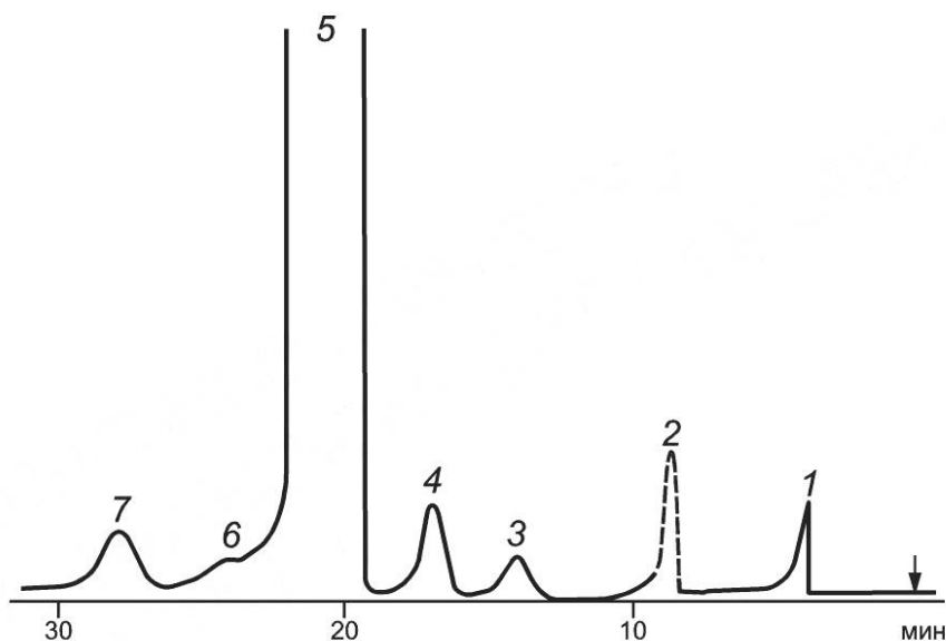
Рисунок 2 — Типовая хроматограмма o -крезола
