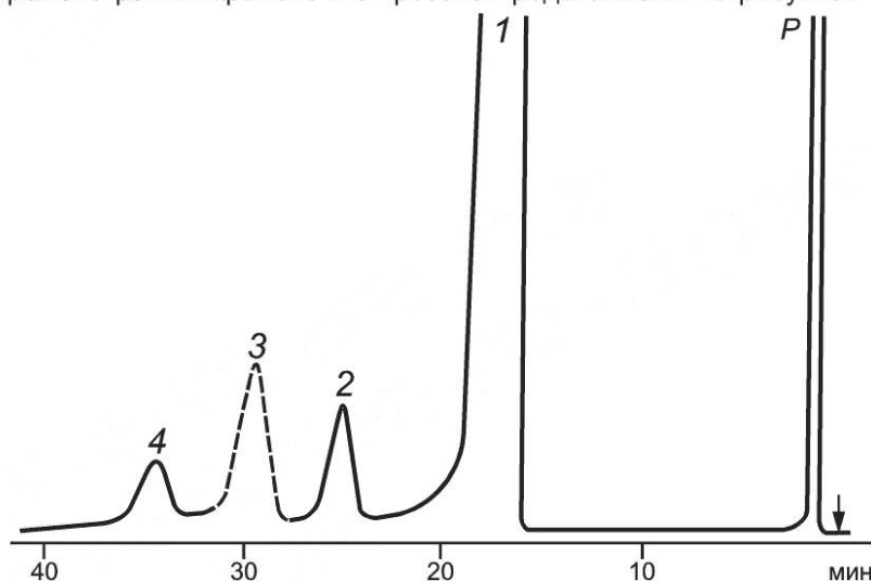
1 — фенол; 2 — o -крезол; 3 — m -крезол (внутренний эталон); 4 — 2,6-ксиленол; P — растворитель
