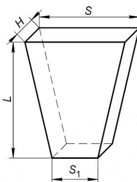
Рисунок 2 — Трапецеидальный двусторонний клин (стеное изделие)
