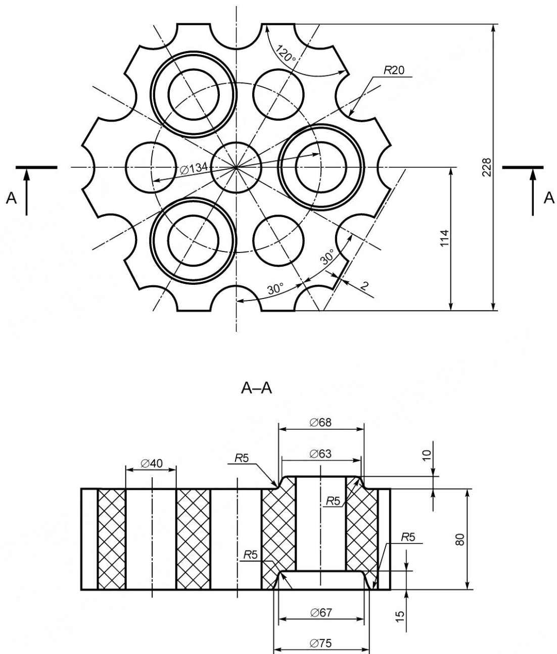
Рисунок 11 — Фасонное изделие номер 80 (насадочное шестигранное)
