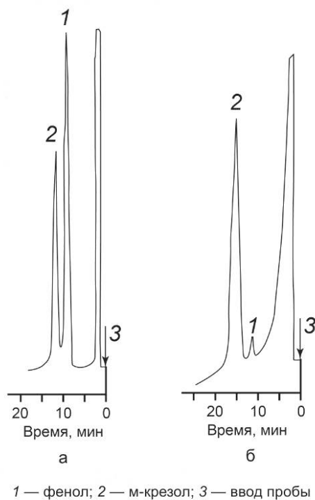
Рисунок 1 — Хроматограмма жидких фенолоформальдегидных смол
