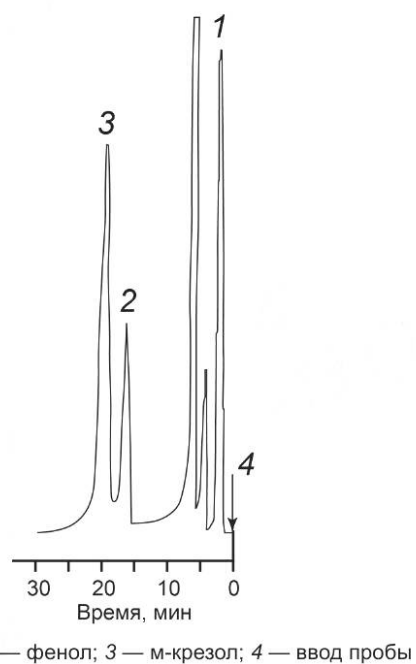
Рисунок 2 — Хроматограмма жидких фенолоформальдегидных смол, содержащих ацетон
