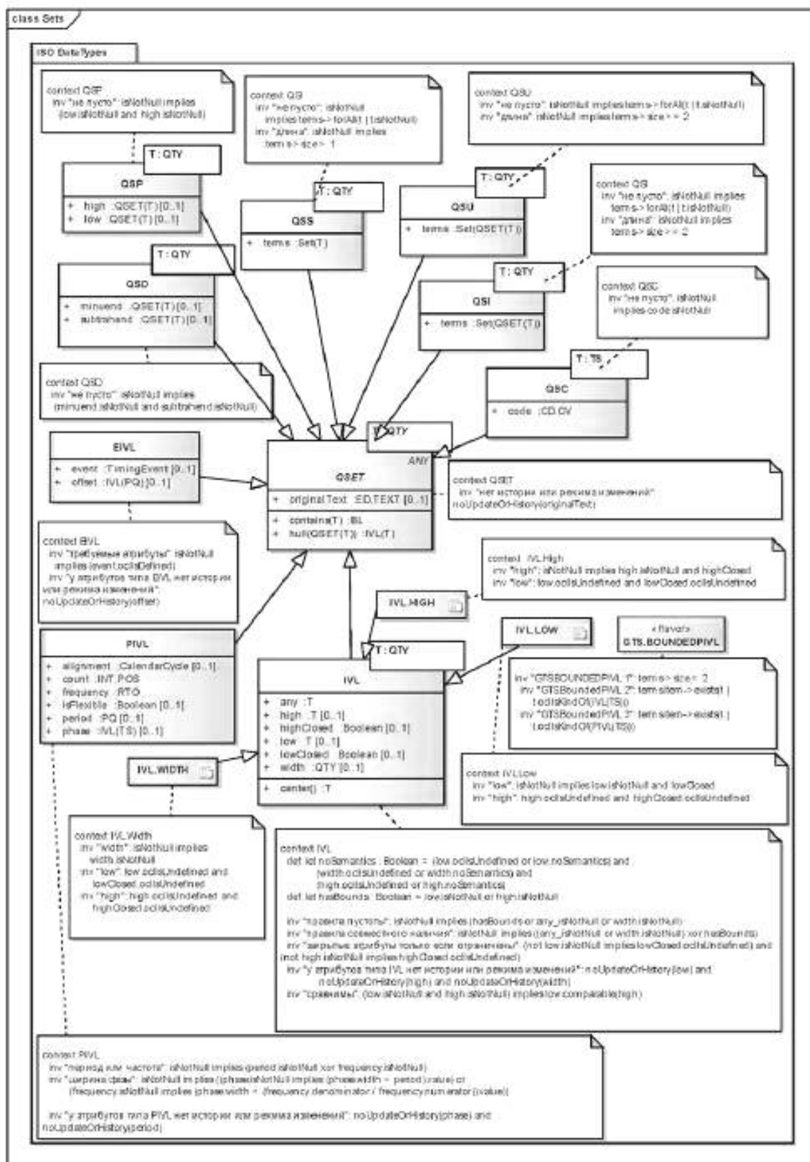
Рисунок 9 — Типы непрерывных множеств
