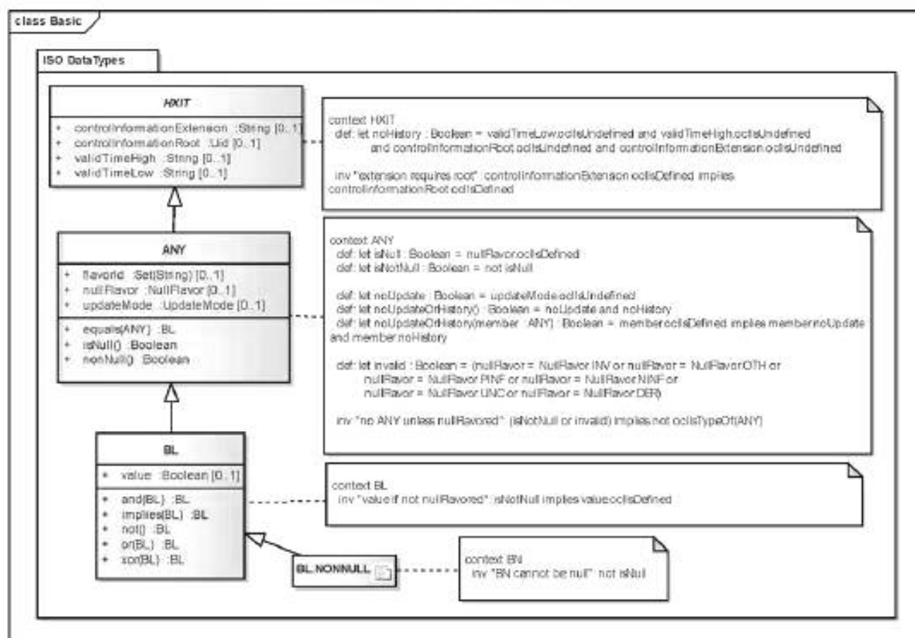
Рисунок 2 — Базовые типы данных
