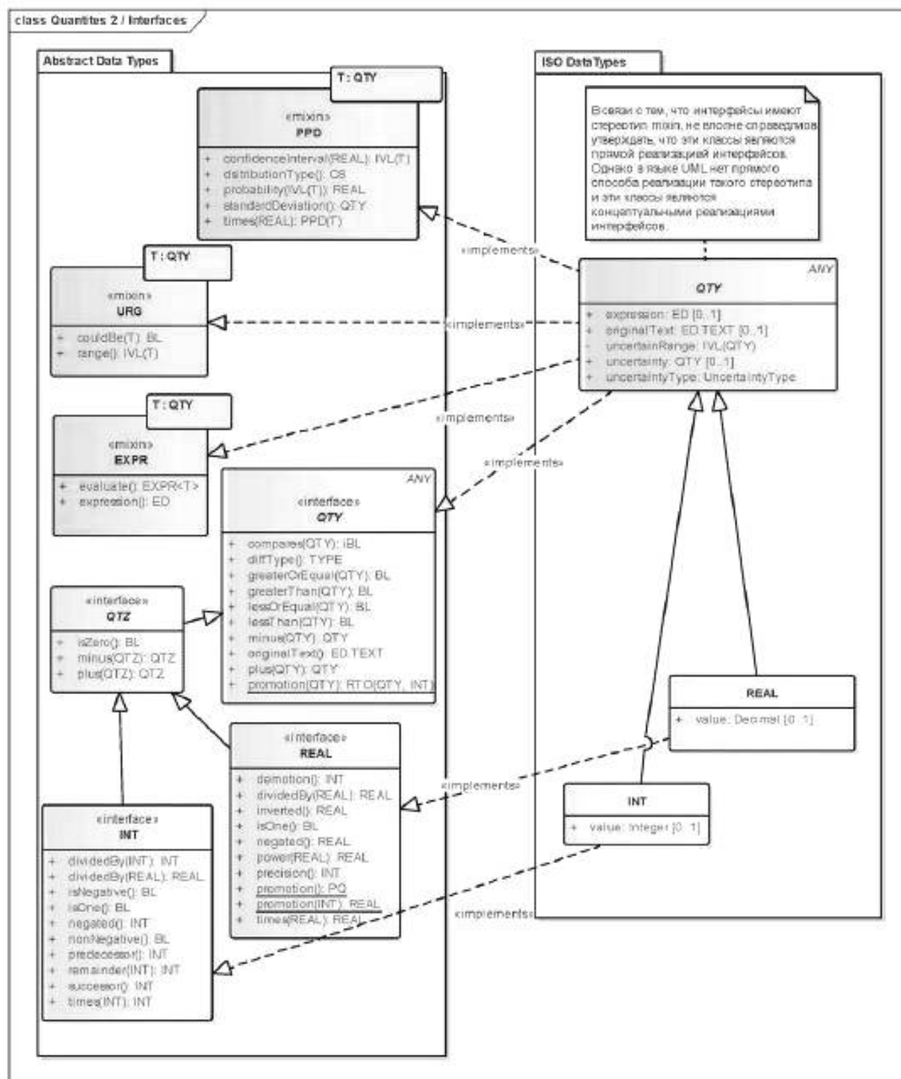
Рисунок D.8 — Отображение базовых количественных типов данных
