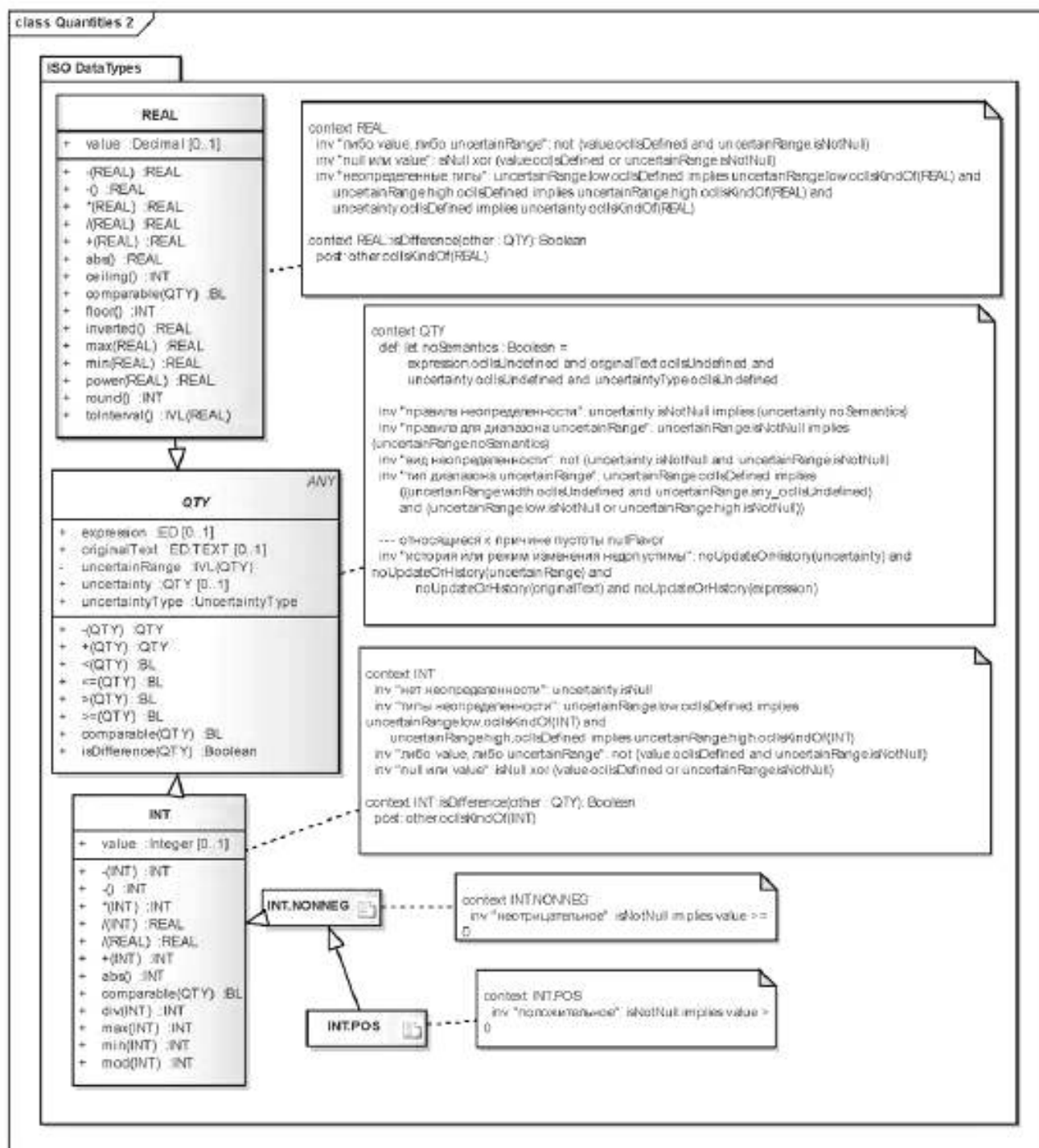
Рисунок 7, лист 1 — Количественные типы данных
