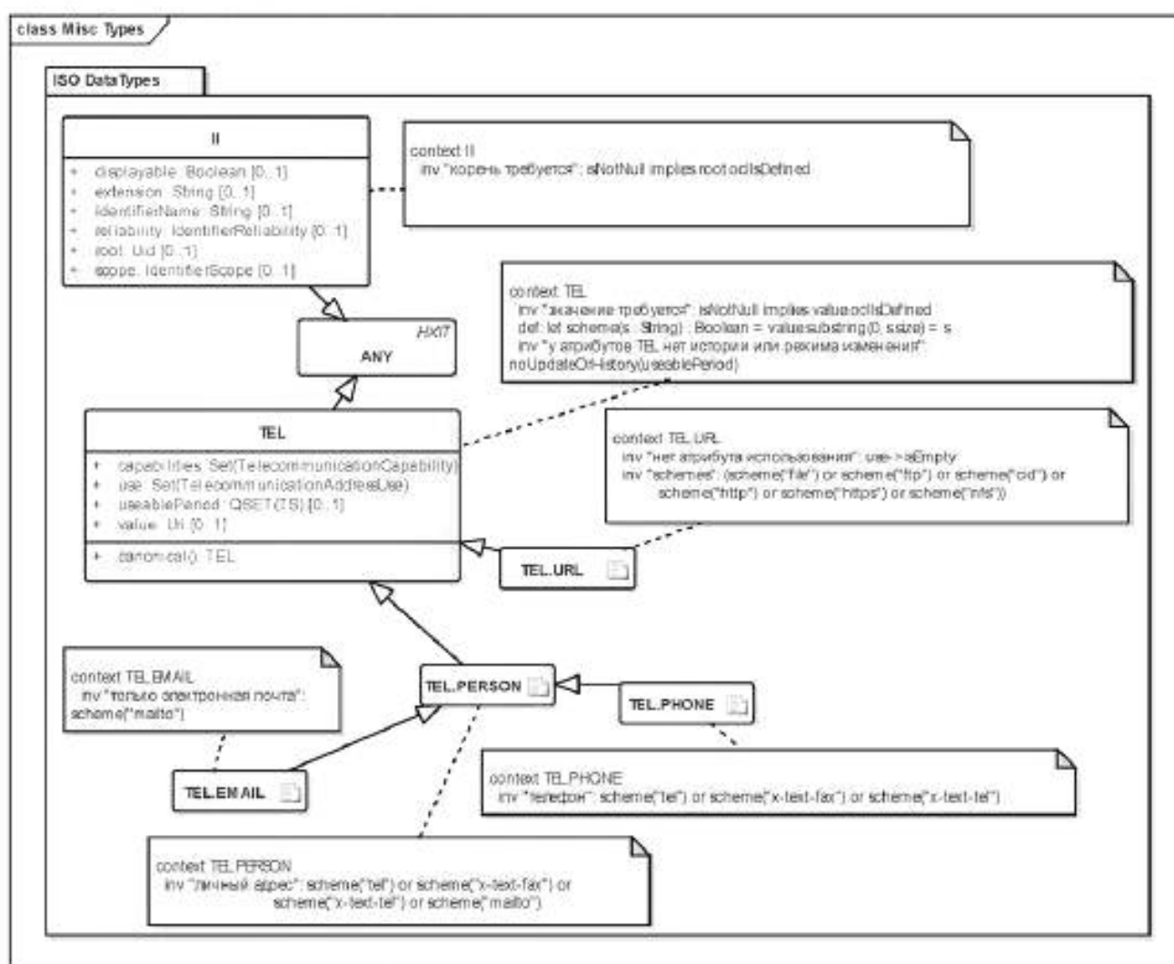
Рисунок 5 — Типы данных идентификации и местонахождения
