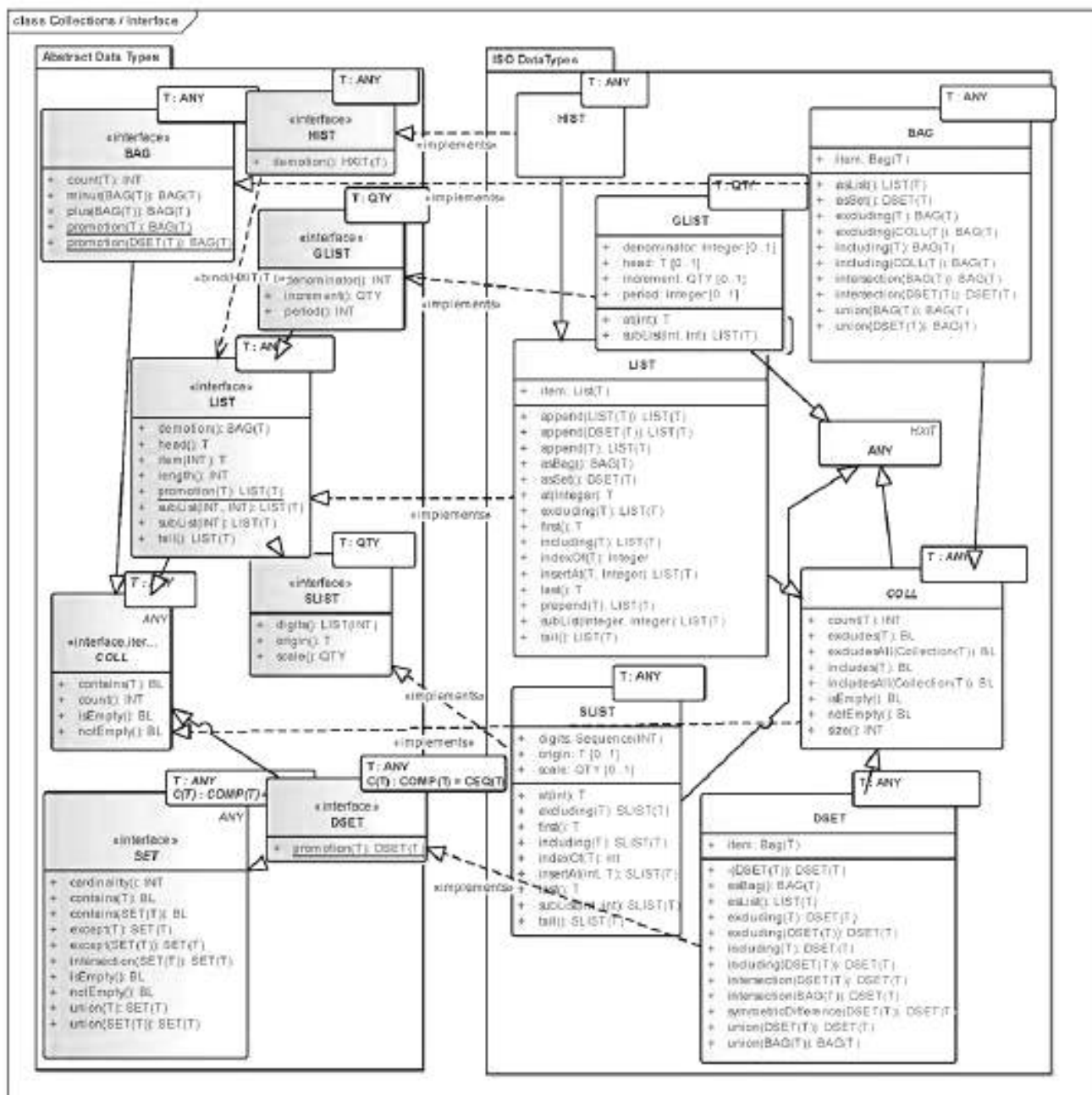
Рисунок D.3 — Отображение типов данных коллекций
