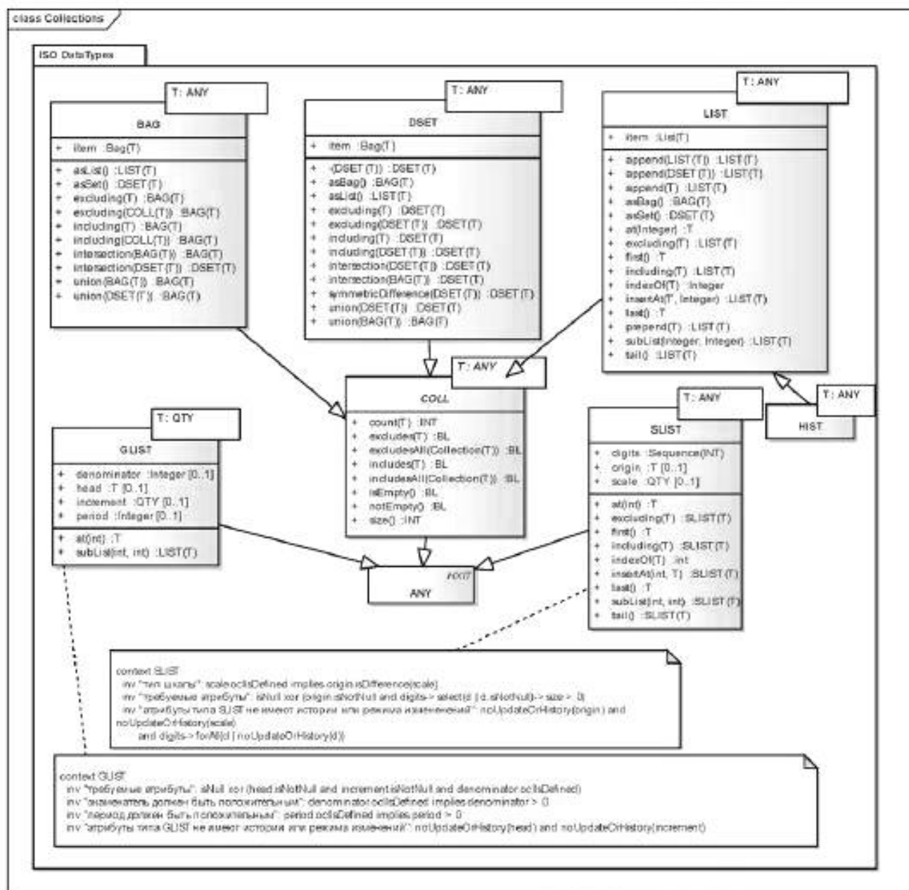
Рисунок 8 — Коллекции типов данных
