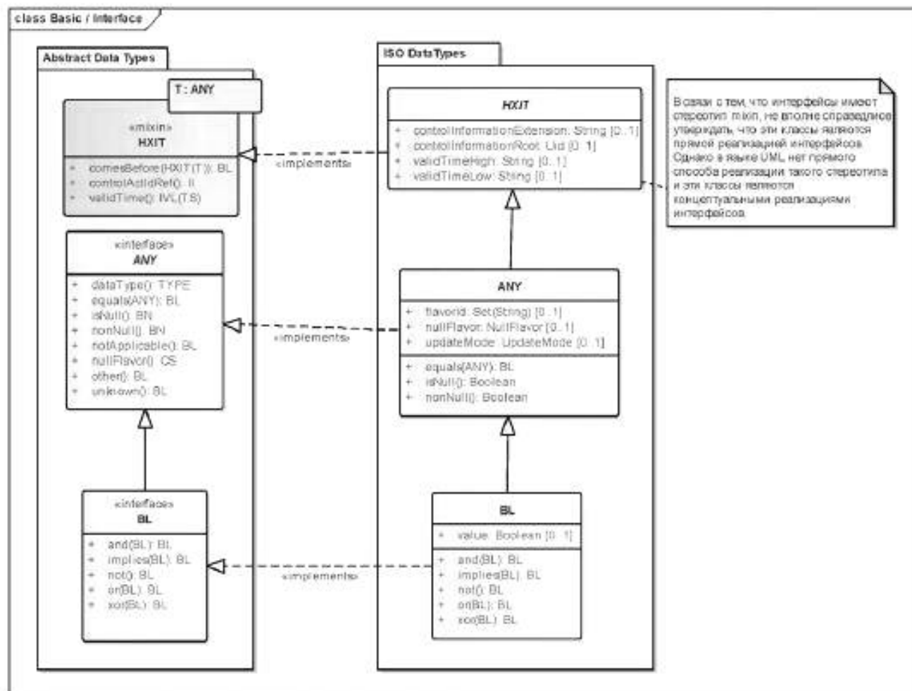
Рисунок D.2 — Отображение базовых типов данных
