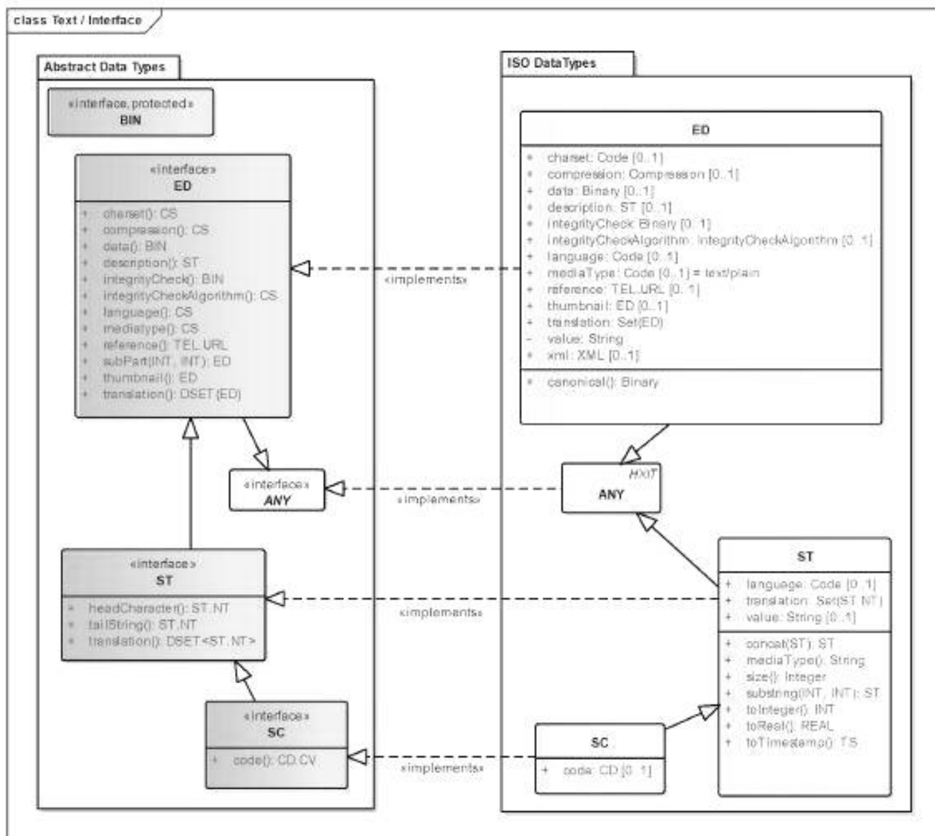
Рисунок D.4 — Отображение текстовых типов данных
