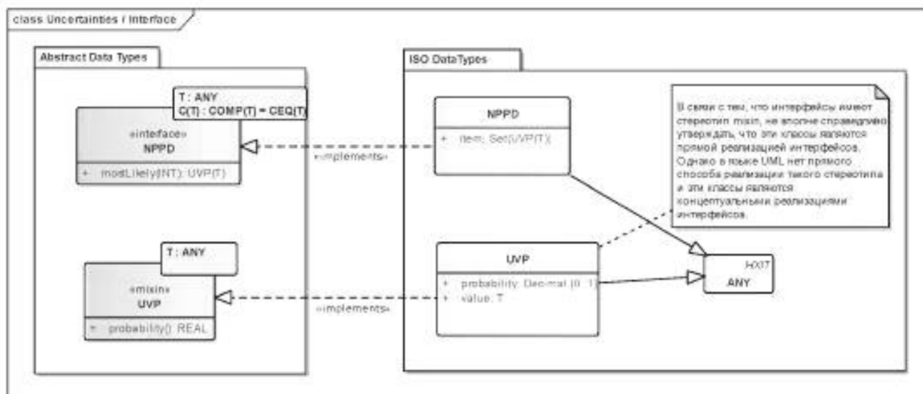
Рисунок D.11 — Отображение типов данных неопределенности
