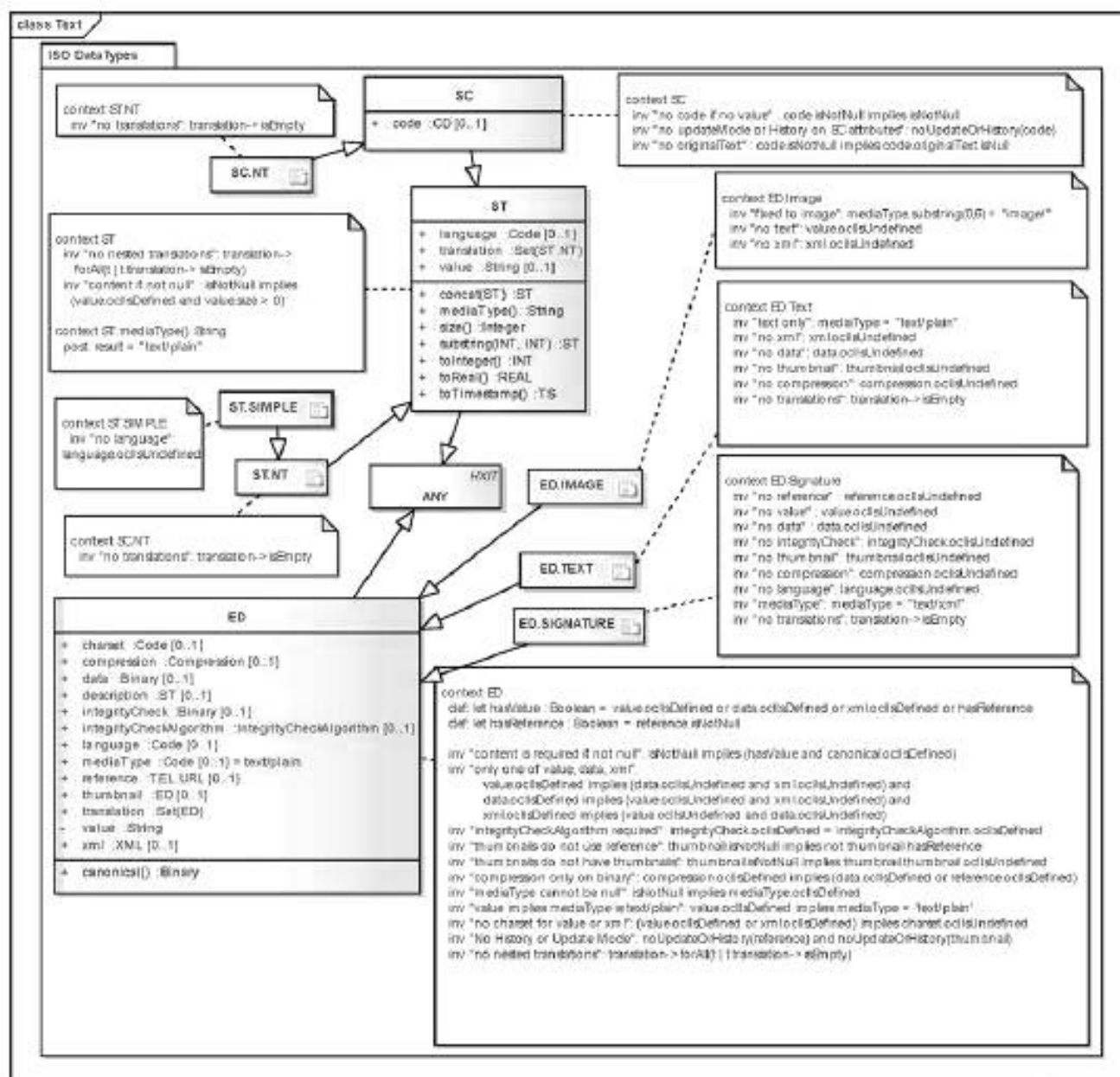
Рисунок 3 — Текстовые и двоичные типы данных
