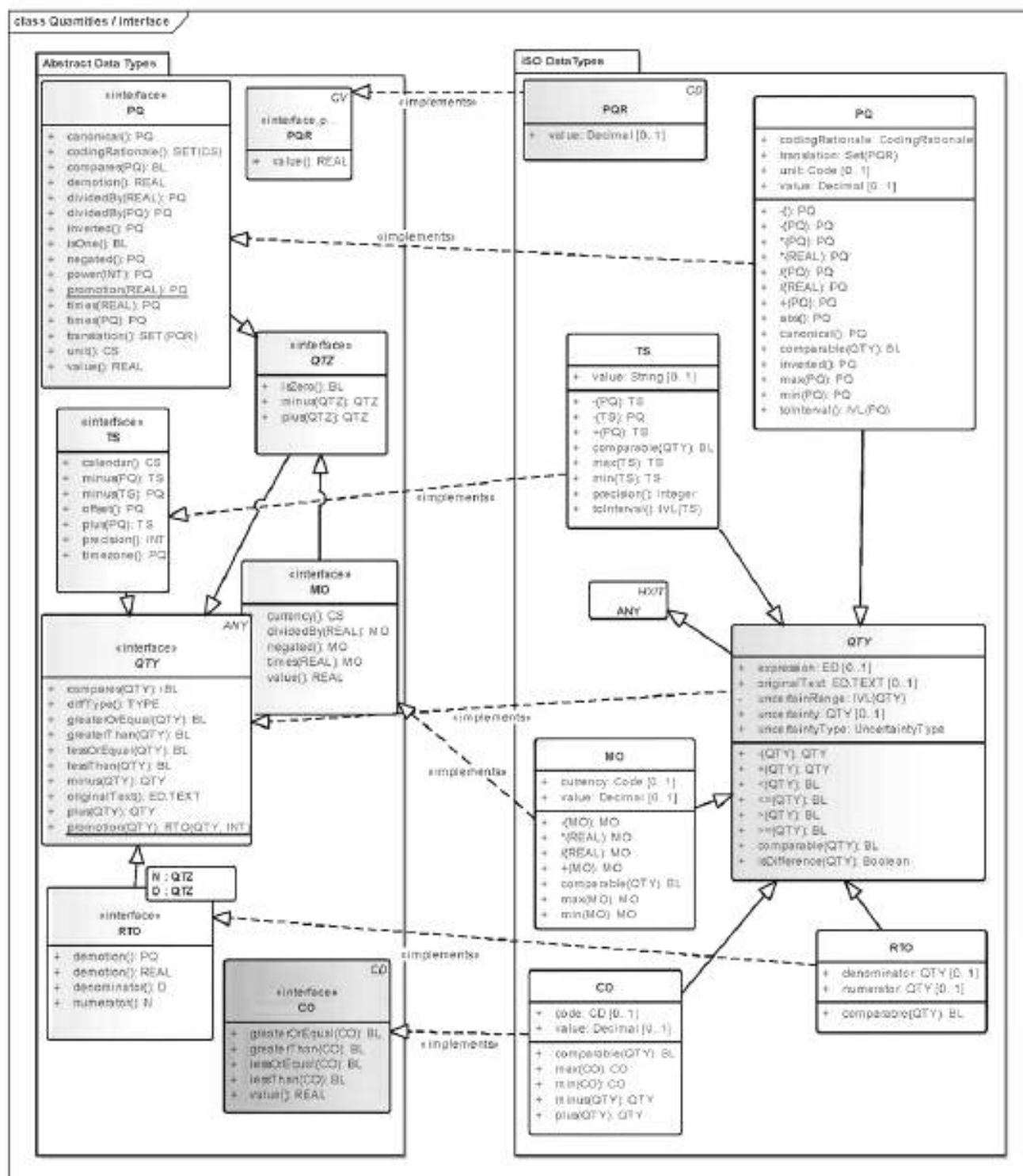
Рисунок D.9 — Отображение количественных типов данных
