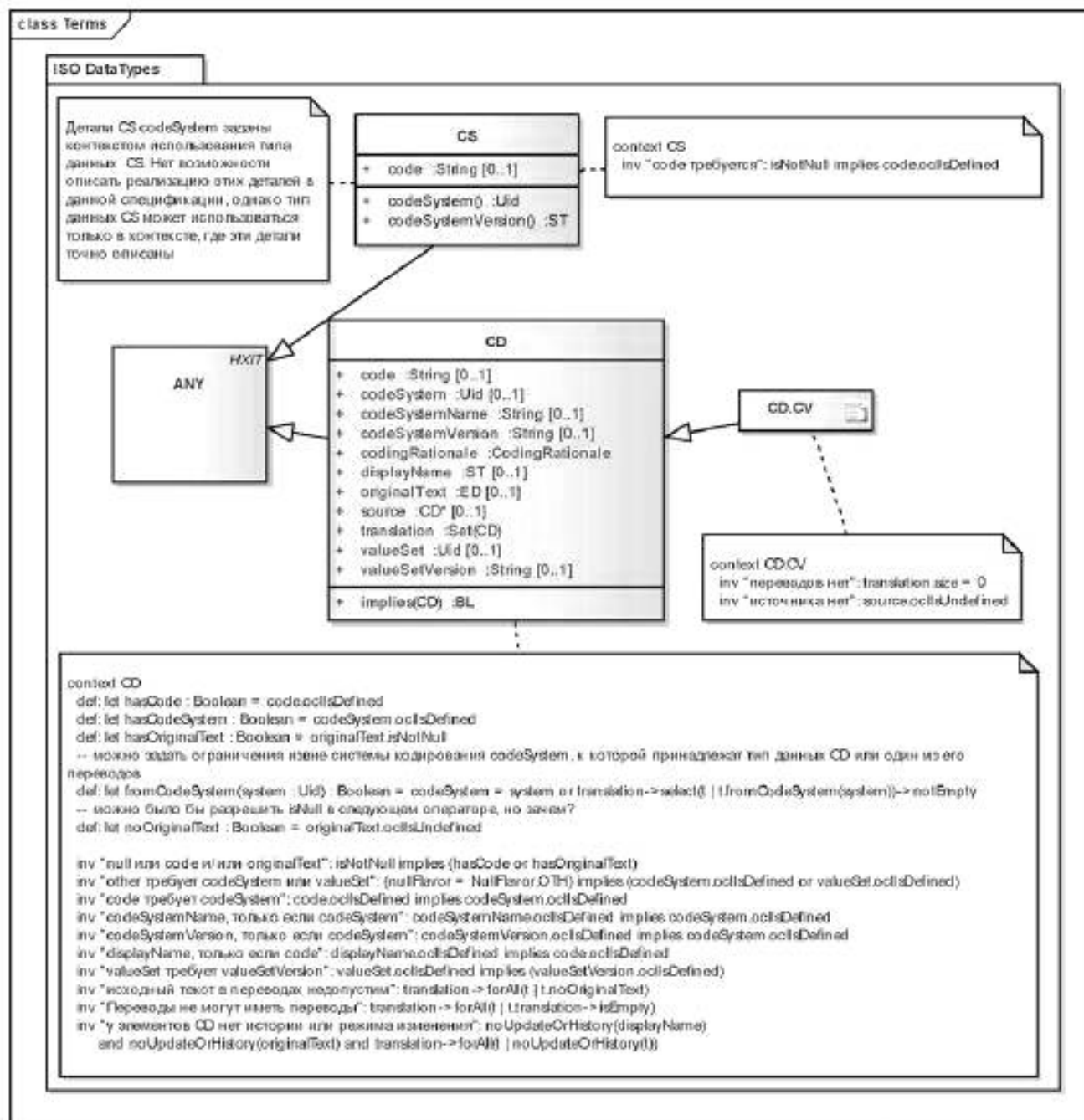
Рисунок 4 — Кодированные типы данных
