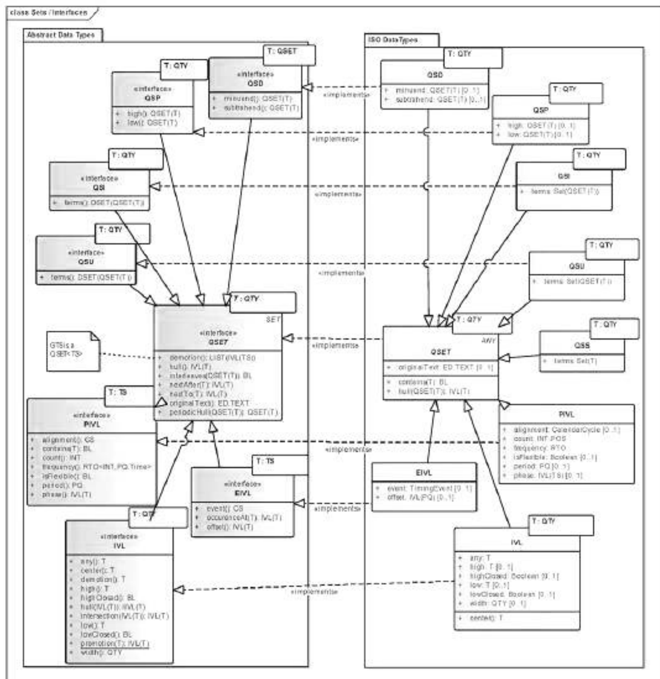
Рисунок D.10 — Отображение множеств количественных типов данных
