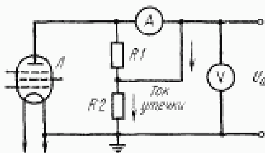
L —лампа, A —амперметр, V —вольтметр, R2 —сопротивление току утечки через охлаждающую воду.
