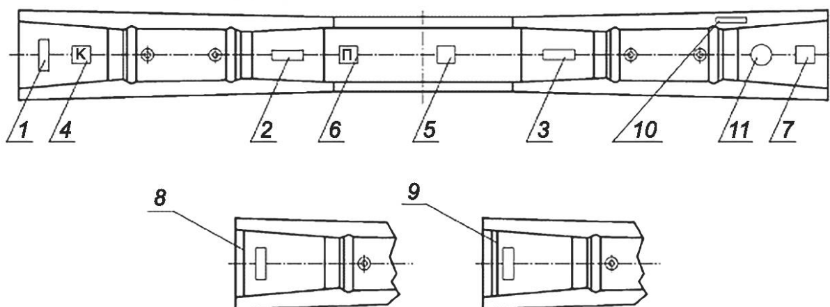
1 — тип шпалы; 2 — товарный знак предприятия-изготовителя; 3 — год изготовления; 4 — обозначение кривой; 5 — знак обращения на рынке; 6 — обозначение шпал исполнения 2; 7 — штамп ОТК и номер партии; 8, 9 — обозначение некондиционной шпалы
