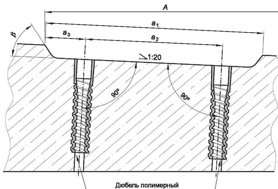
б — для шурупно-дюбельного крепления
