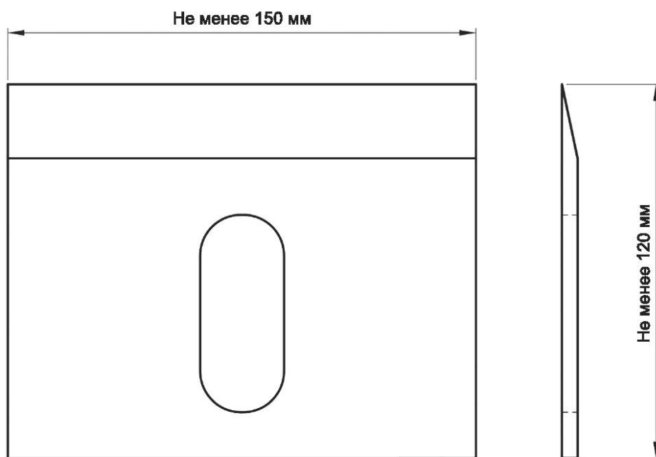
Рисунок 9 — Металлический шаблон
