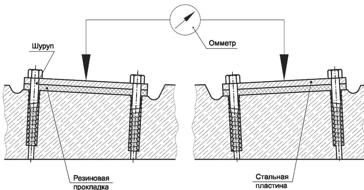
Рисунок 18 — Схема измерения электрического сопротивления шпалы
