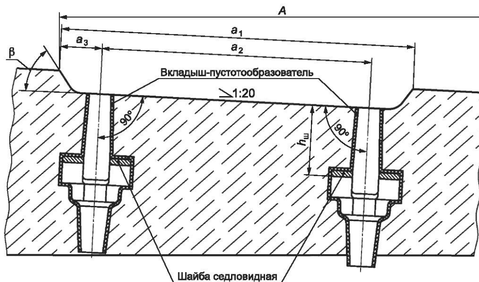
а — для болтового крепления
