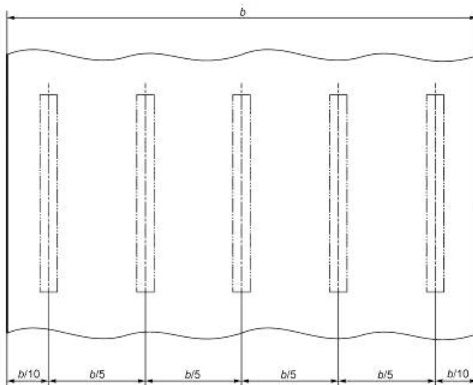
Рисунок 3 — Участки вырубания образцов
