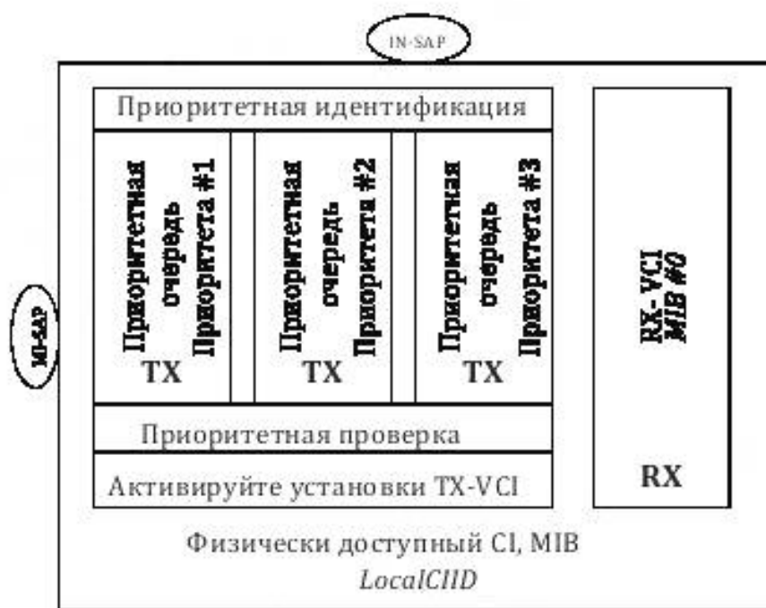
Рисунок 8 — Приоритетные очереди CI и виртуальные интерфейсы связи
