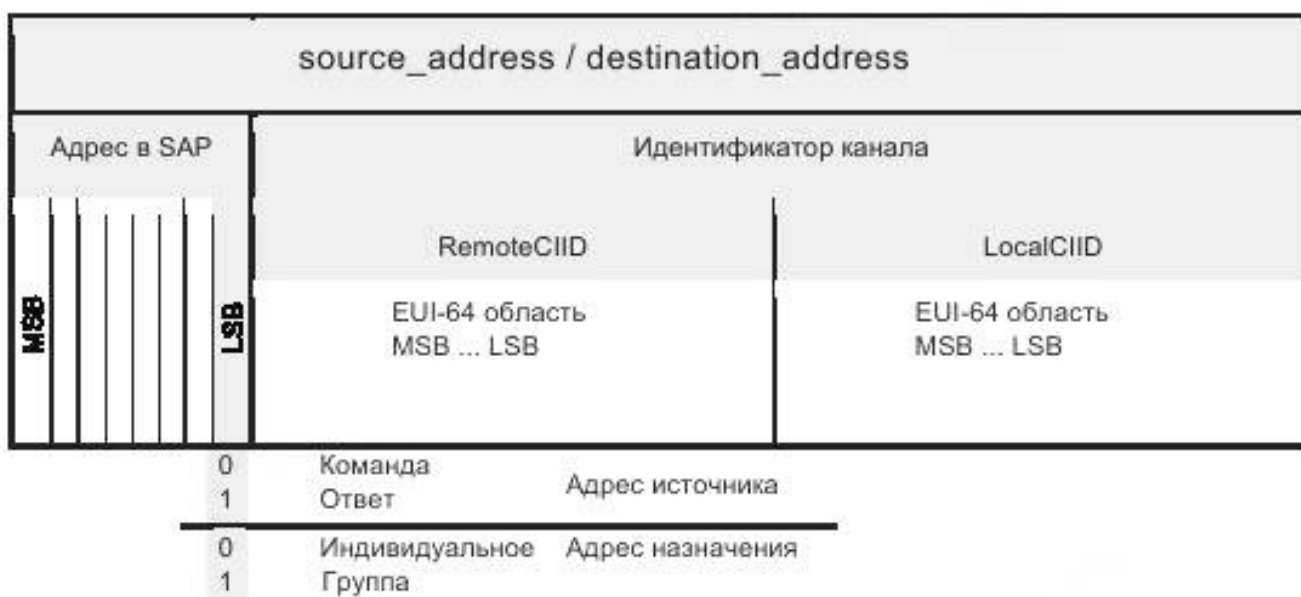
Рисунок 9 — Формат адреса источника и адреса назначения В SAP
