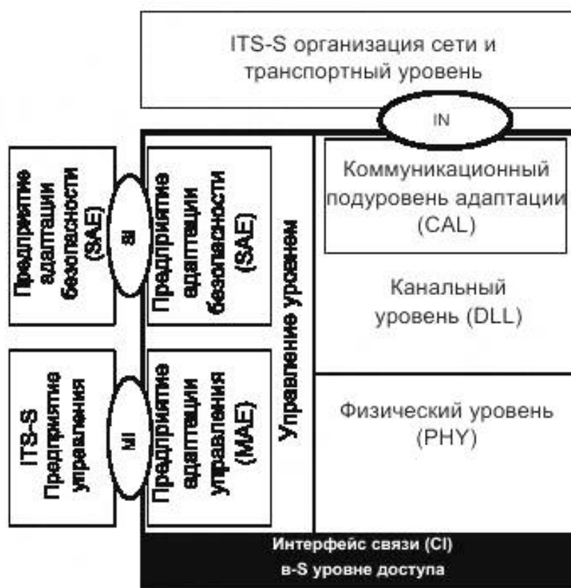
Рисунок 2 — Архитектура
