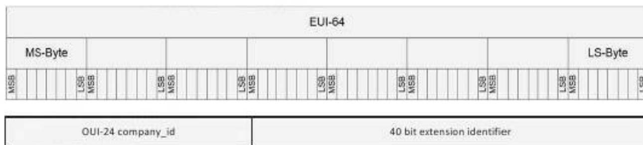
Рисунок С.1 — EUI-64 формат
