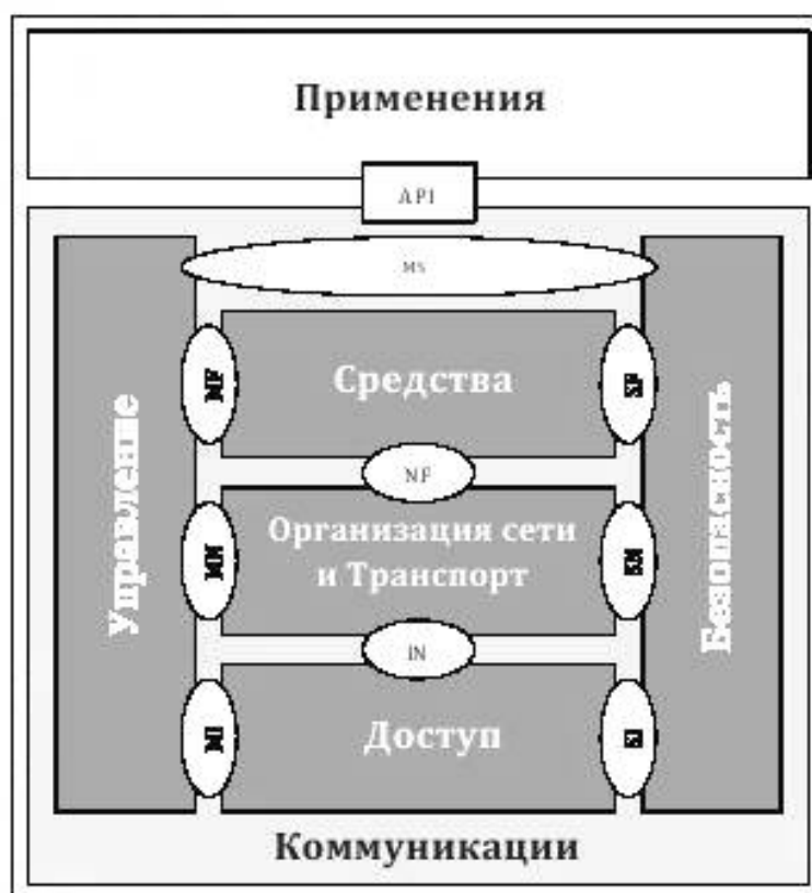
Рисунок 1 — ИТС станционная справочная архитектура с названными интерфейсами
