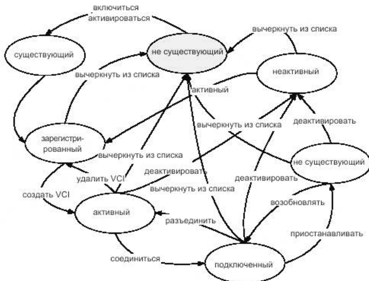
Рисунок 4 — Конечный автомат CI
