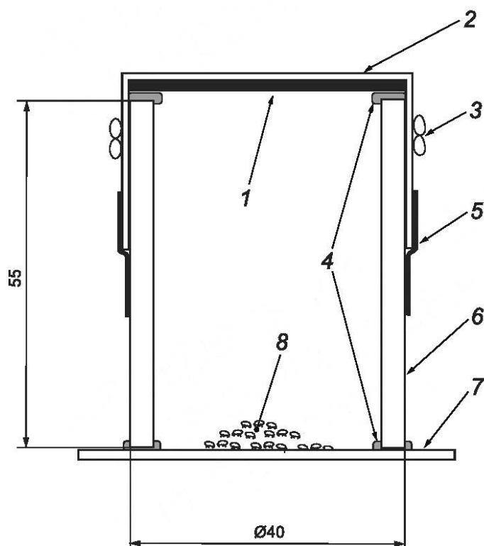
1 — испытуемая проба; 2 — пищевая пленка; 3 — резинка; 4 — термоклей; 5 — клейкая лента; 6 — стеклянная трубка В; 7 — бумажный фильтр; 8 — клещевая среда
