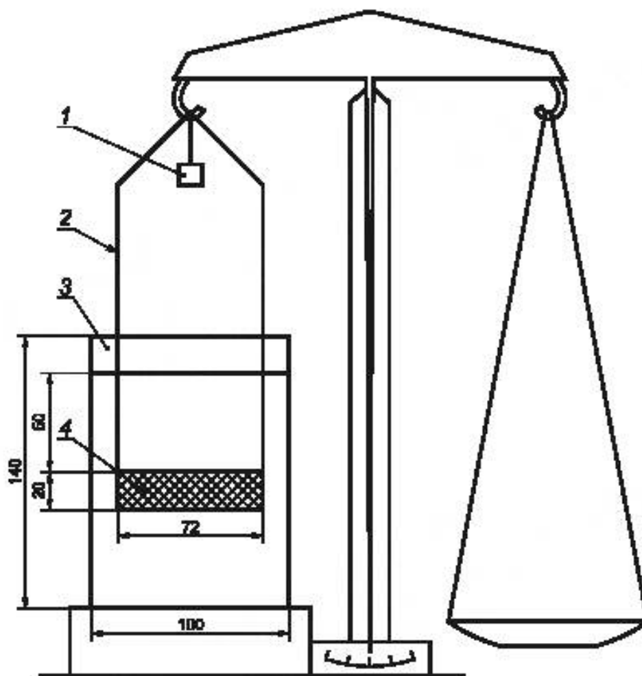
1 — компенсирующий груз; 2 — медная проволока; 3 — стакан вместимостью 800 см 3 ; 4 — корзина из металлической сетки с размером отверстий 5 × 5 мм
