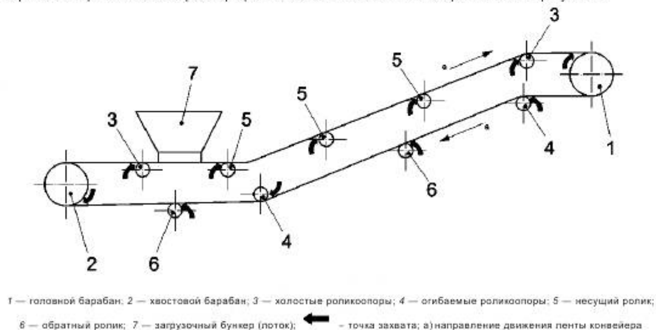
Рисунок В.1 — Расположение точек захвата
