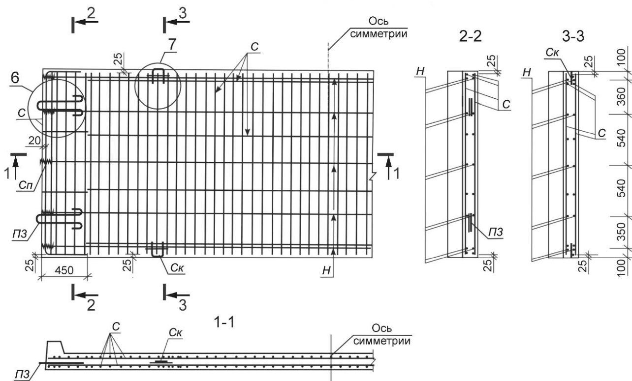
Рисунок Б.4 — Схема армирования плиты PBB55.20
