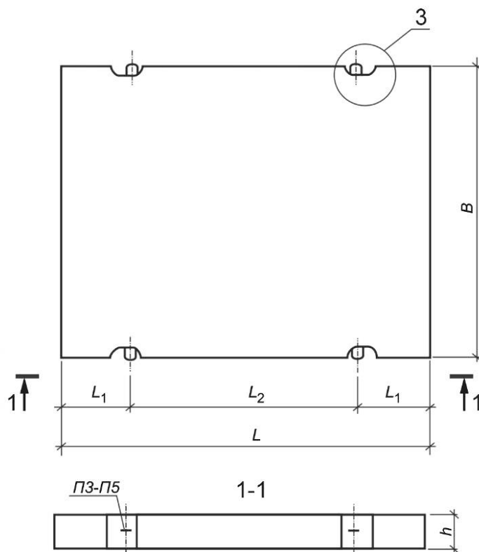
Рисунок А.3 — Плиты П35.28, П30.18, П18.18, П18.15
