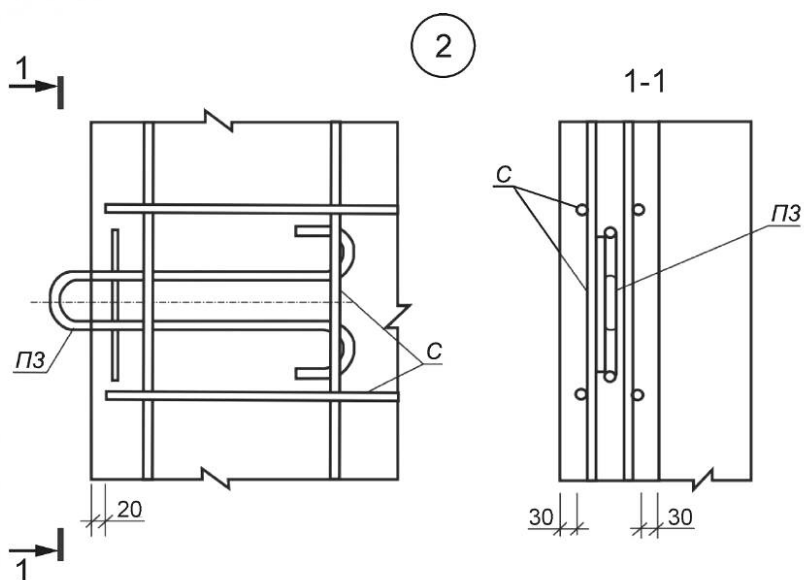
Рисунок В.8 — Армирование плиты. Узел 2
