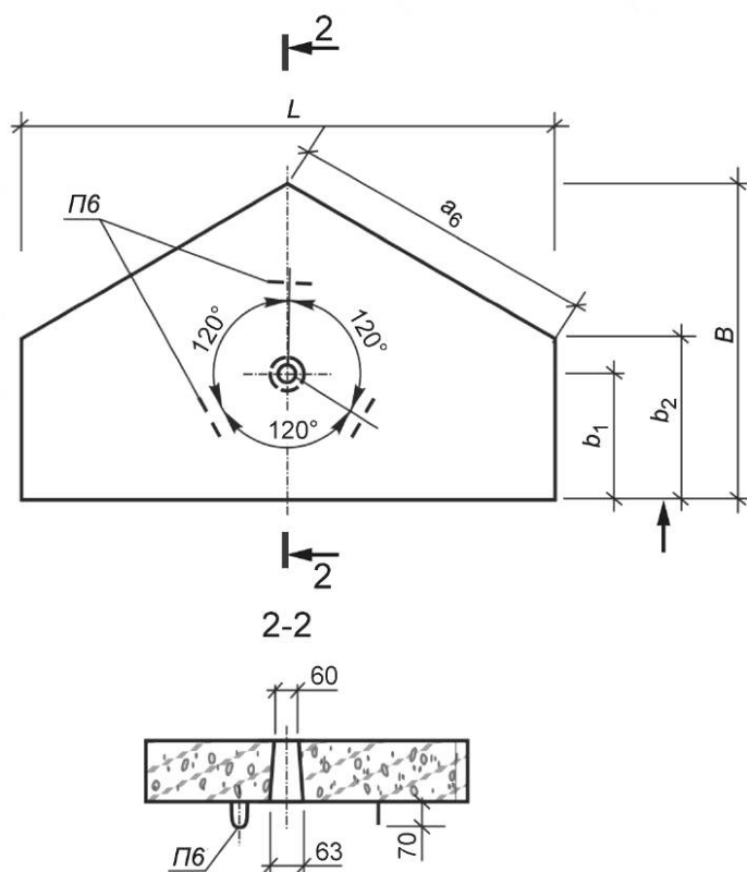
Рисунок А.11 — Плита ППШ
