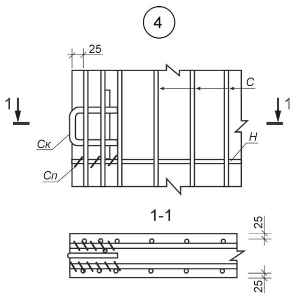
Рисунок Б.9 — Узел армирования 4
