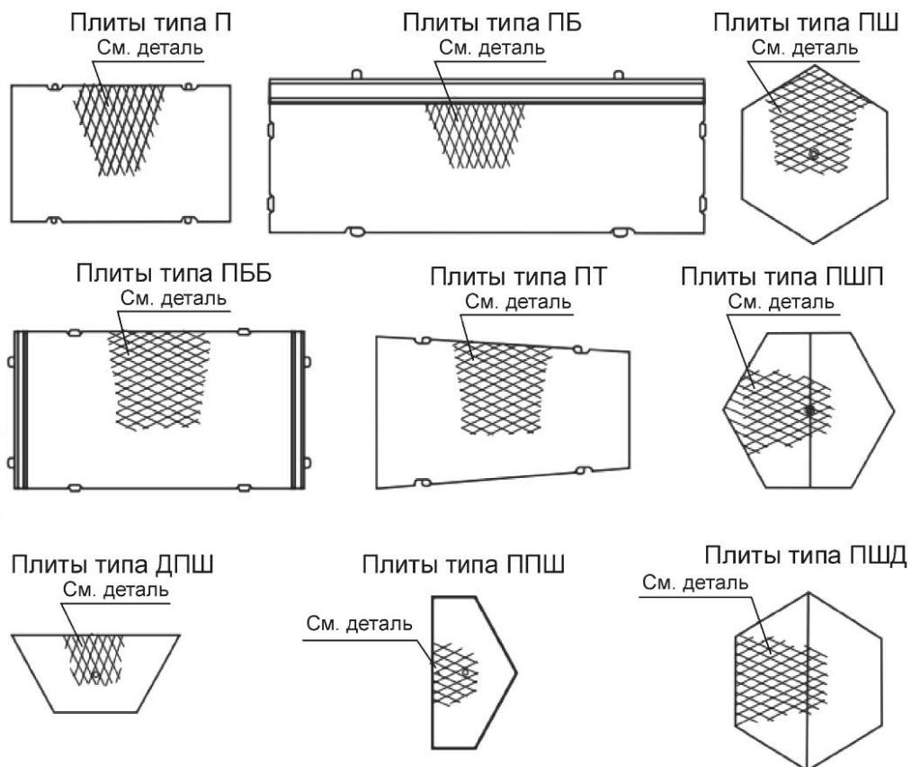
Деталь рифления на рабочей поверхности плит
