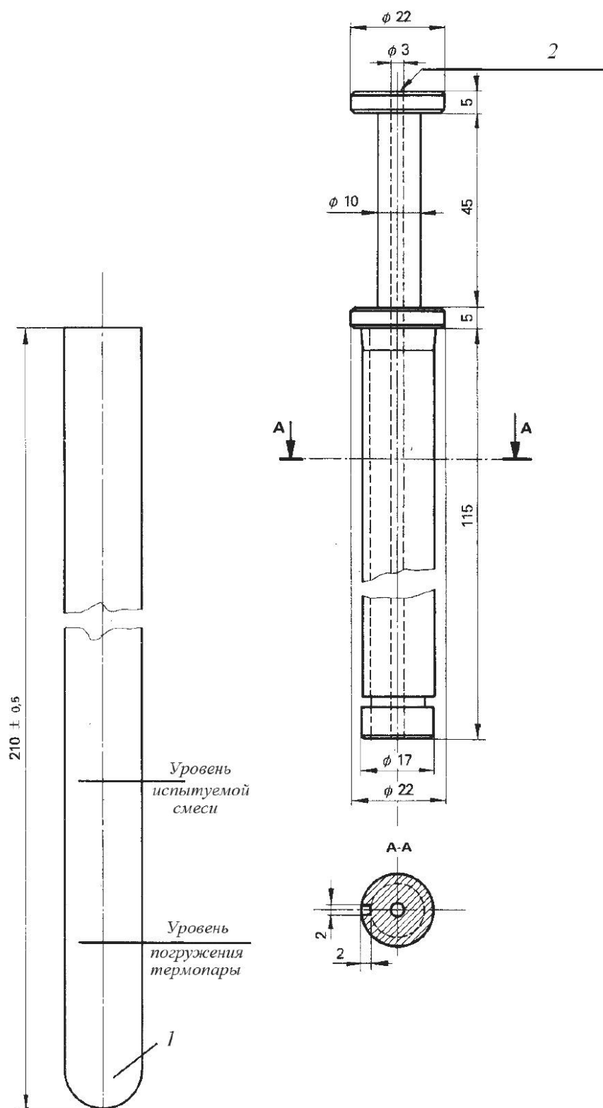
Рисунок 1 – Пример приспособления для центрирования термопары
