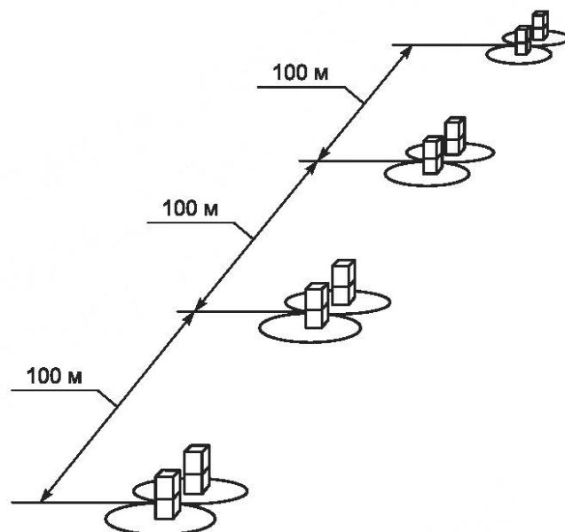
Рисунок Е.1 — Размещение испытательного оборудования
