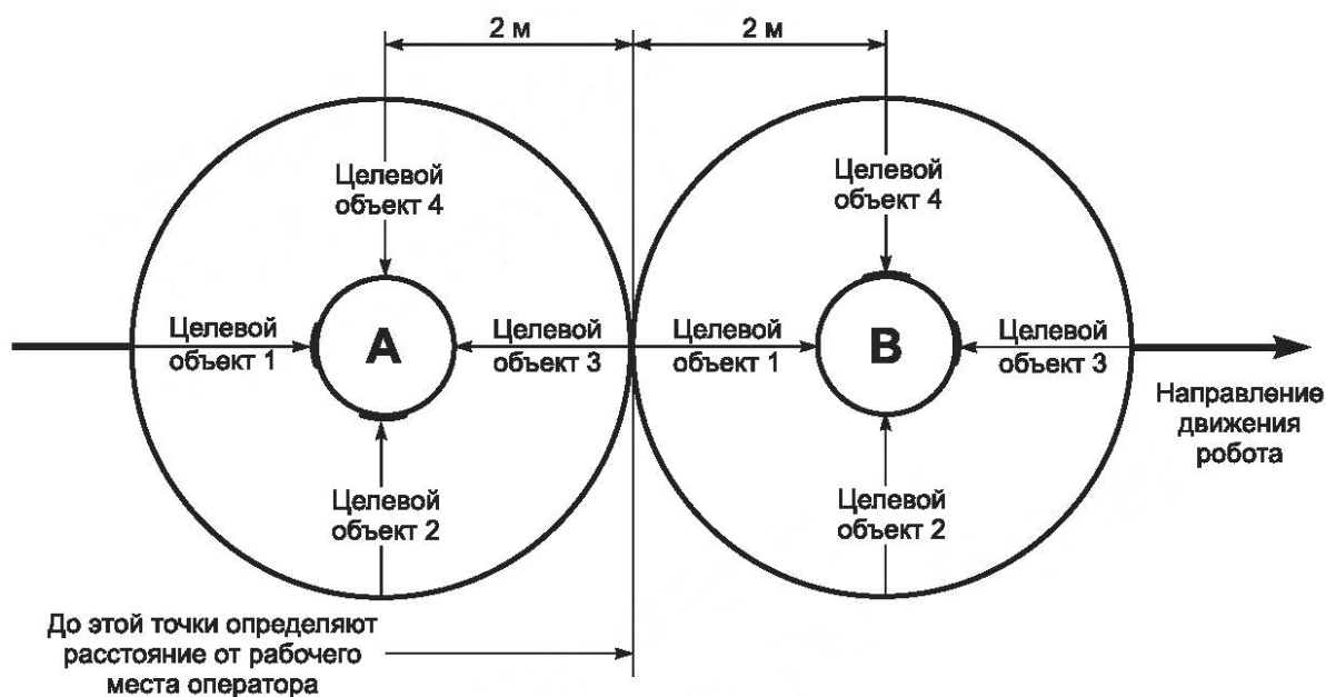
Рисунок Е.2 — Схема испытательного поста
