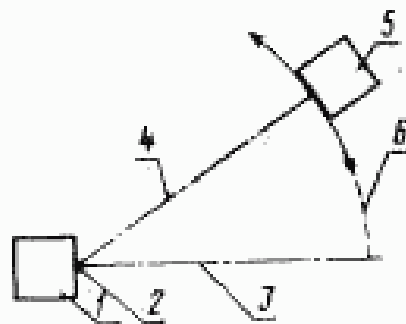
1—рентгеновская трубка; 2—действительное фокусное пятно рентгеновской трубки; 3—ось рабочего пучка рентгеновского излучения; 4—оптическая ось блока детектирования; 5—блок детектирования; 6—направление вращения блока детектирования
