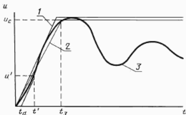
Построение огибающей ПВН, определяемого двумя параметрами
