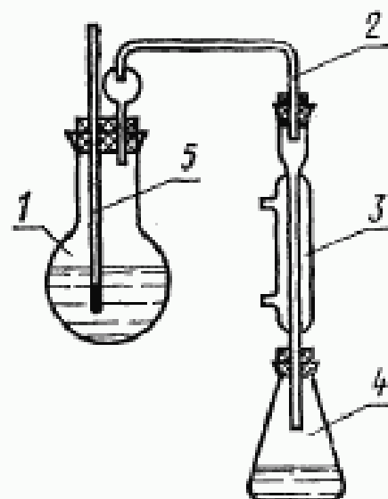
Установка для дистилляции мышьяка
