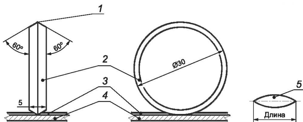
1 — острый край; 2 — индентор; 3 — покрытие; 4 — основание; 5 — форма отпечатка
