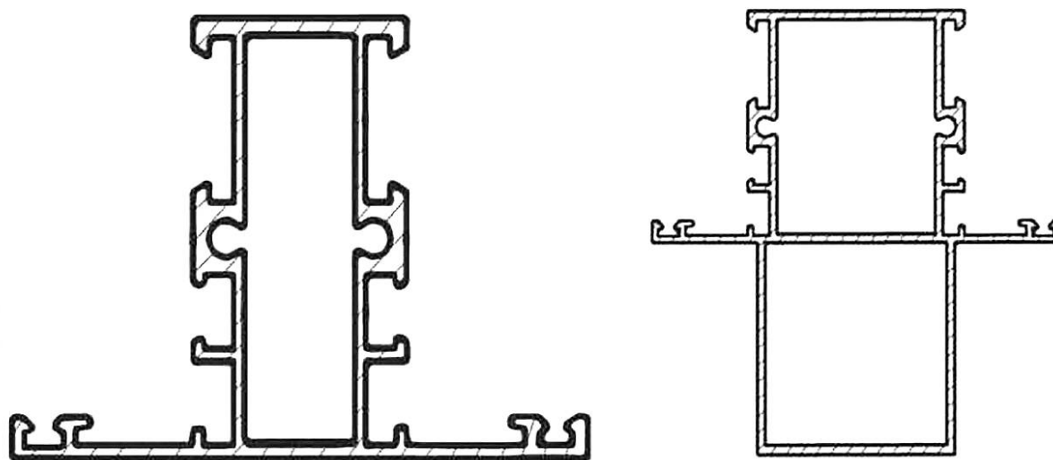
Рисунок 2 — Полый профиль
