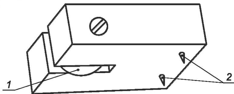
1 — индентор; 2 — опоры
