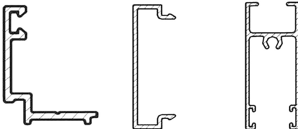
Рисунок 1 — Сплошной профиль
