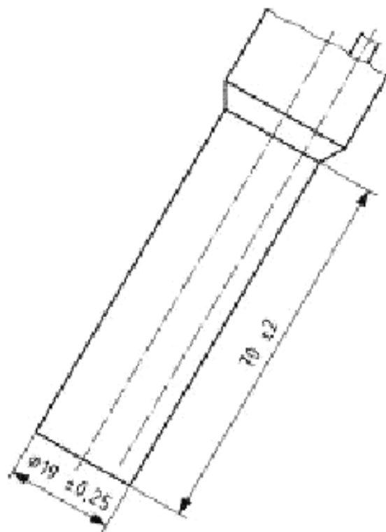
Рисунок 3 — Сопло
