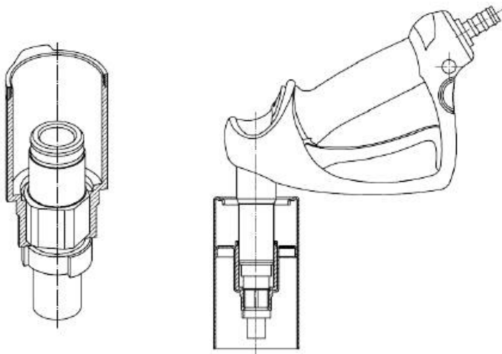
Рисунок А.1 — Пример герметичной системы дозаправки
