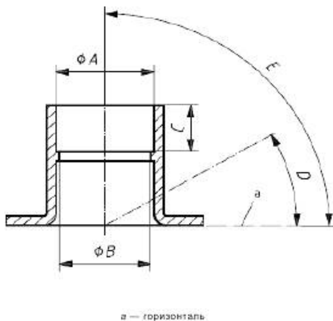
Рисунок 1 — Заливная горловина
