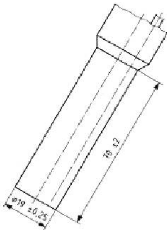
Рисунок 3 — Сопло
