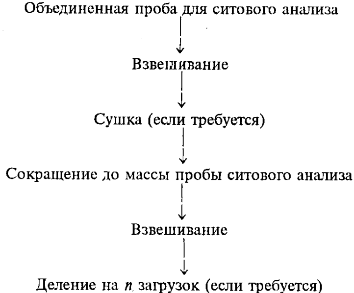
Рисунок 1 — Схема подготовки объединенной пробы к ситовому анализу
