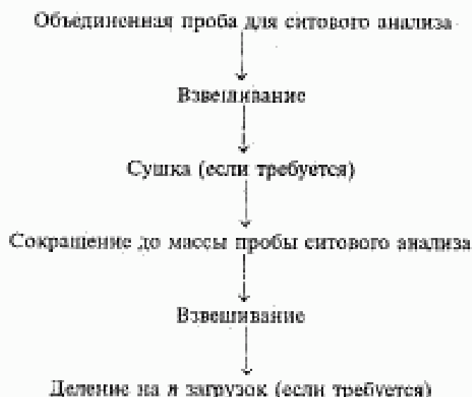
Рисунок 1 — Схема подготовки объединенной пробы к ситовому анализу
