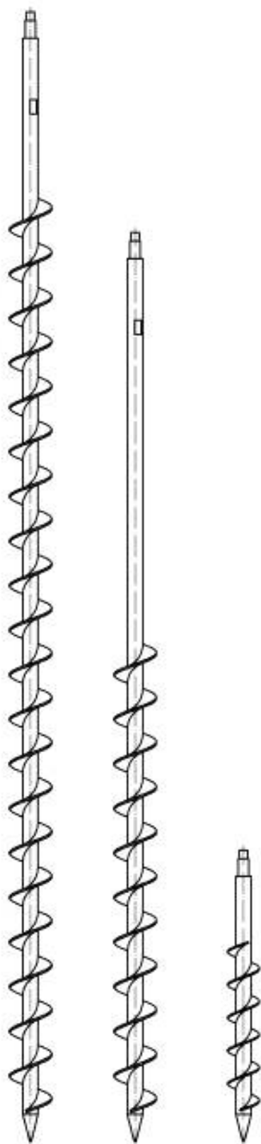
Рисунок С.28 — Шнековые буры с диаметрами от 36 до 100 мм — Категория метода отбора проб С
