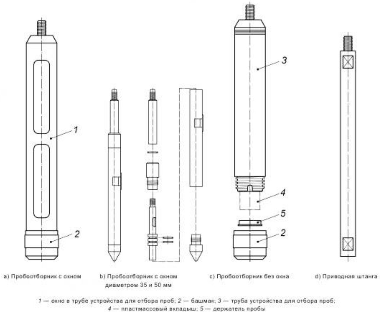
Рисунок С.23 — Устройства для отбора проб с боковым окном и без окна
