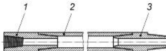
1 — оконечная муфта буровой штанги; 2 — труба штанги; 3 — замыкающий болт
