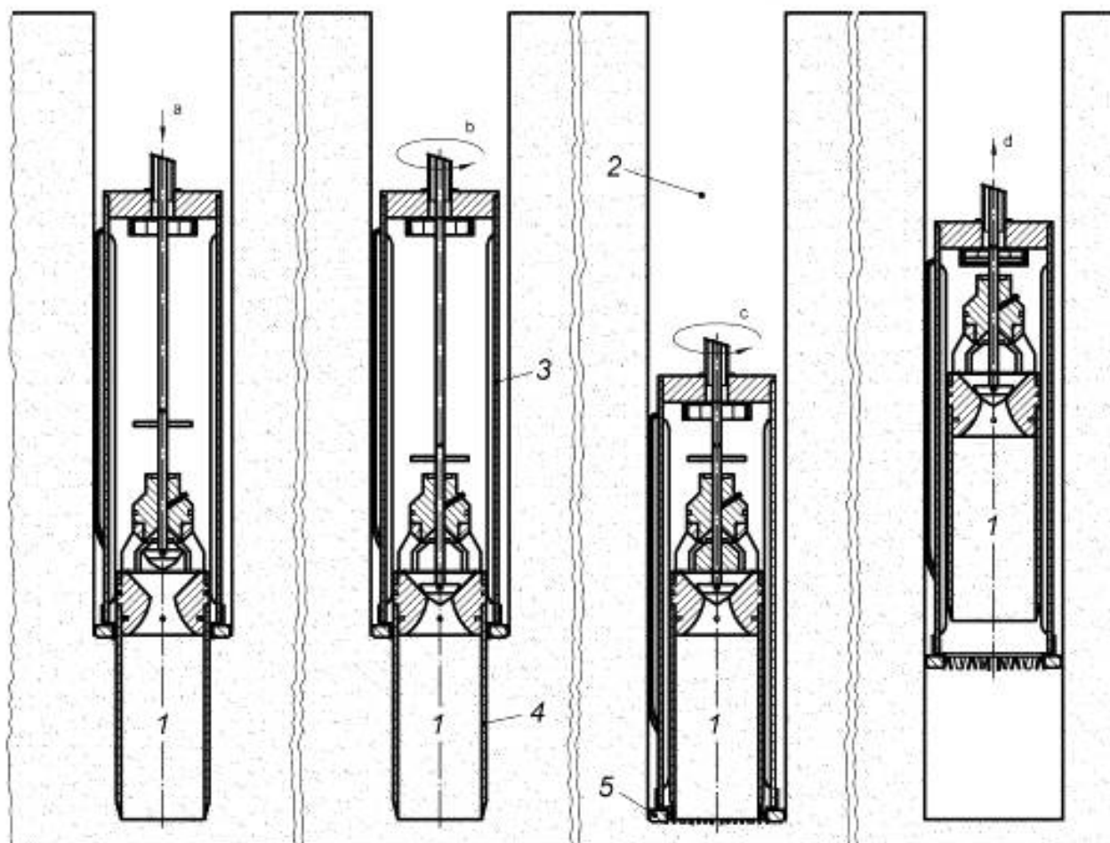
1 — проба грунта в пробоотборнике; 2 — скважина диаметром 300 мм; 3 — колонковая труба; 4 — труба отбора пробы; 5 — режущие зубья
