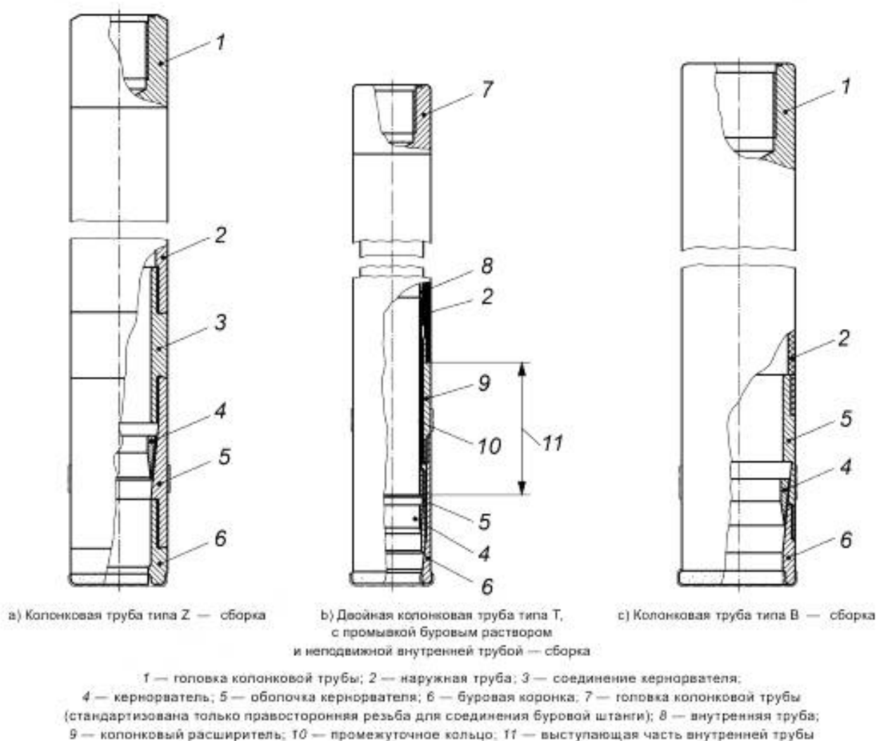
Рисунок С.4 — «Метрическая» серия колонковых труб согласно ИСО 3552-1
