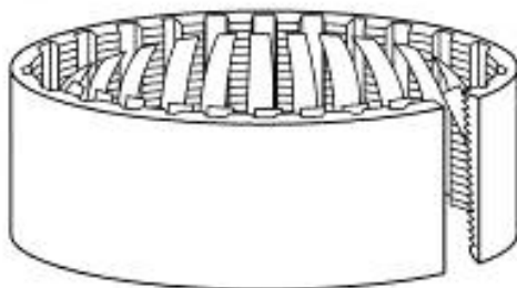
е) С прорезями, зубчатый изнутри и с пальцами корзиночного типа
