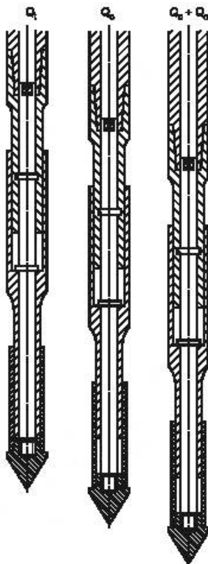
Рисунок 3 — Наконечник M2 (конус с кожухом, муфта трения)
