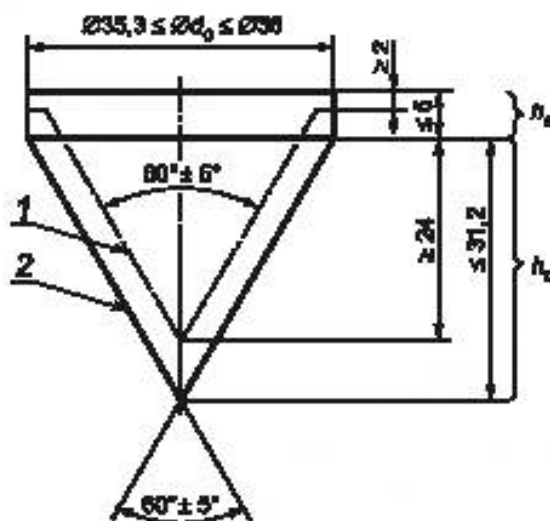
1 — минимальная форма конуса после износа; 2 — максимальная форма конуса
