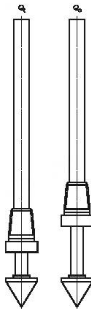
Рисунок 4 — Наконечник M4 (простой конус)
